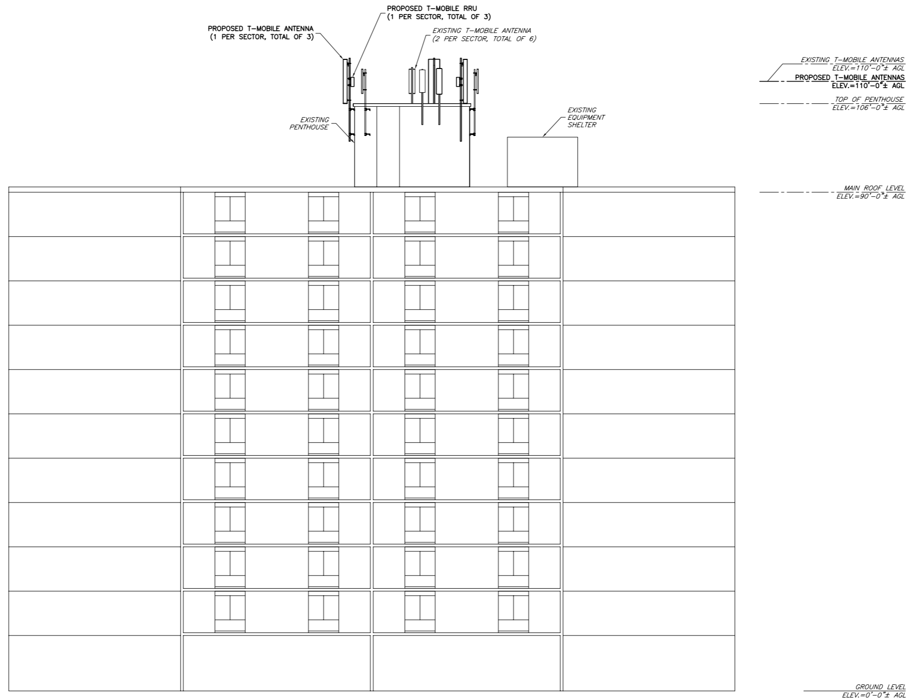
1 ELEVATION C-2 SCALE: 1"=8'
