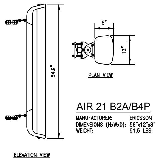
1 TYP. ANTENNA DETAIL A-3 SCALE: N.T.S.
