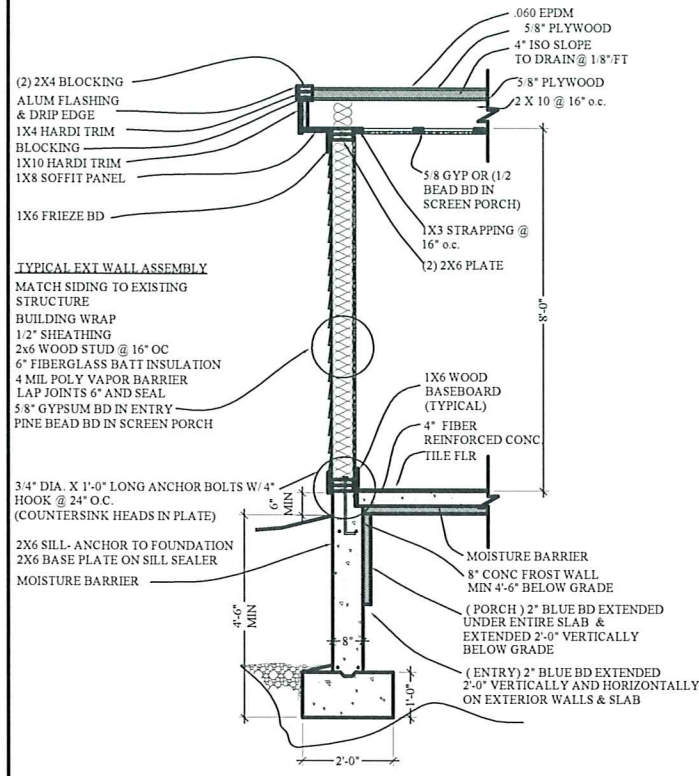
1 WALL SECTION SCALE: 1/2"=1'
