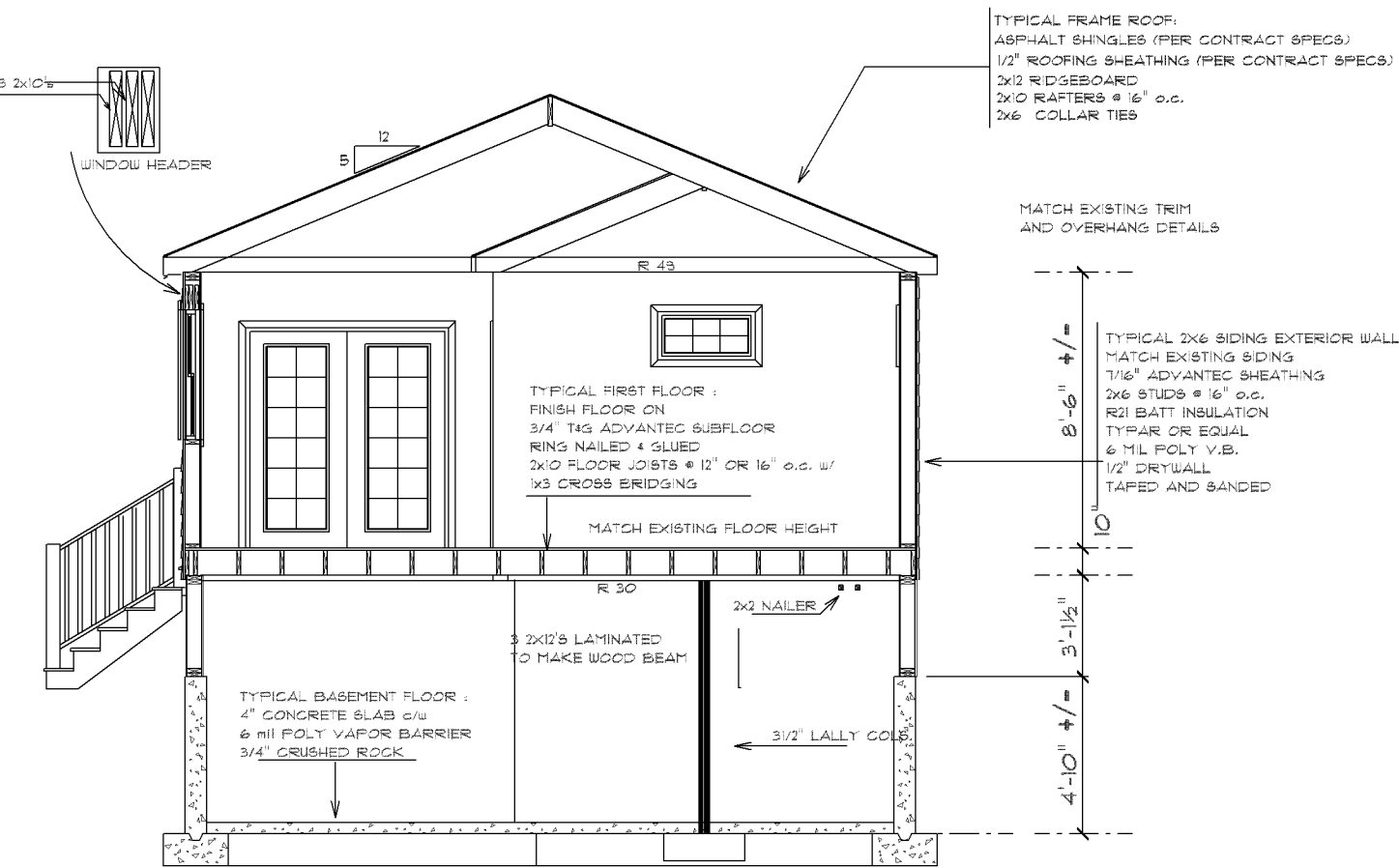
CROSS SECTION A-A SCALE: 1/4" = 1'-0"
