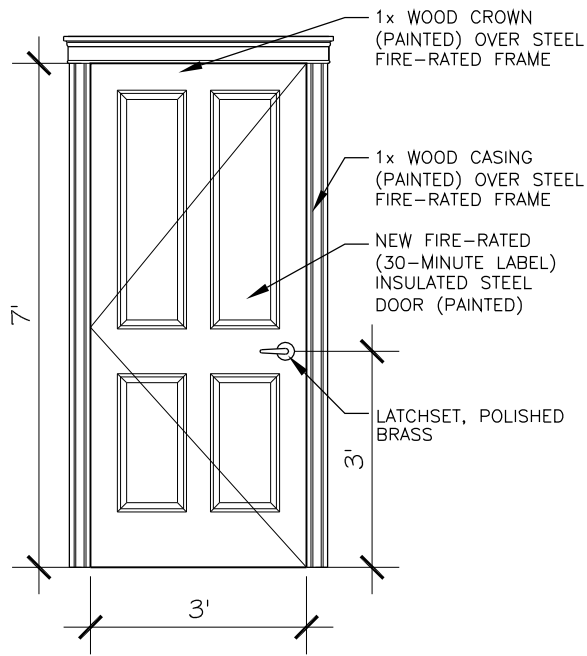
DOOR TYPE A
