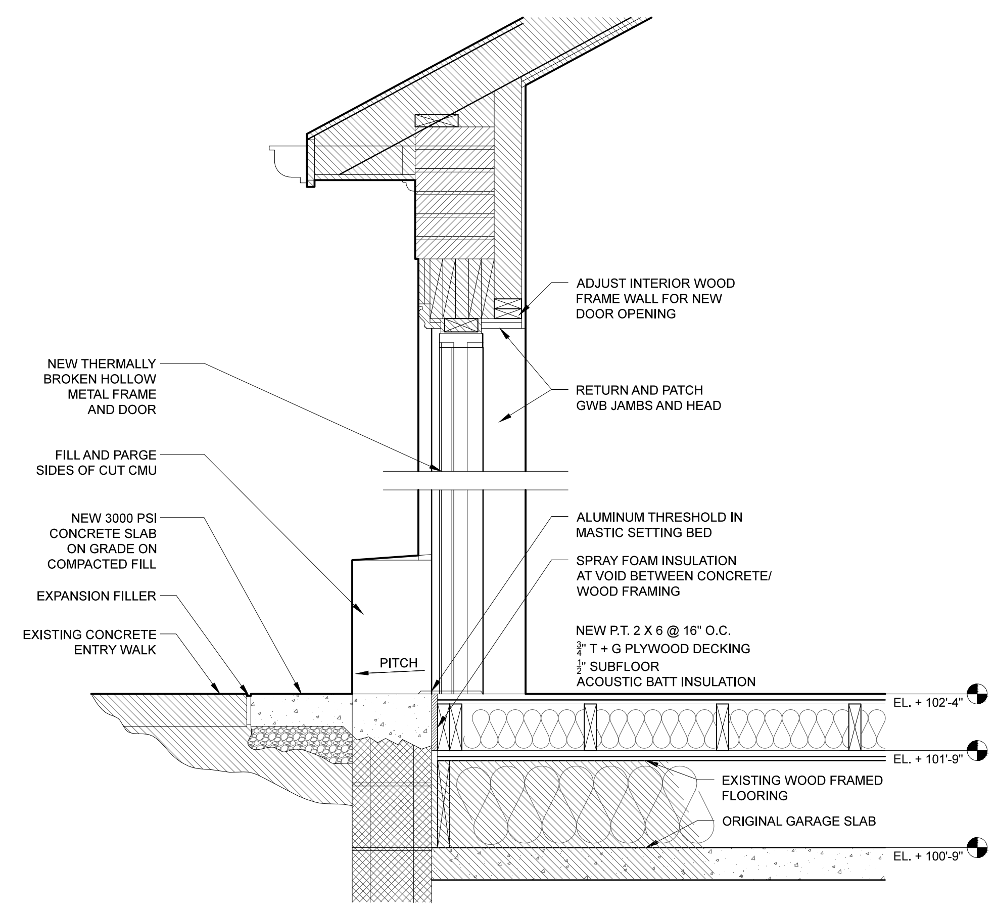
3 Wall Section SCALE: 1" = 1'-0"
