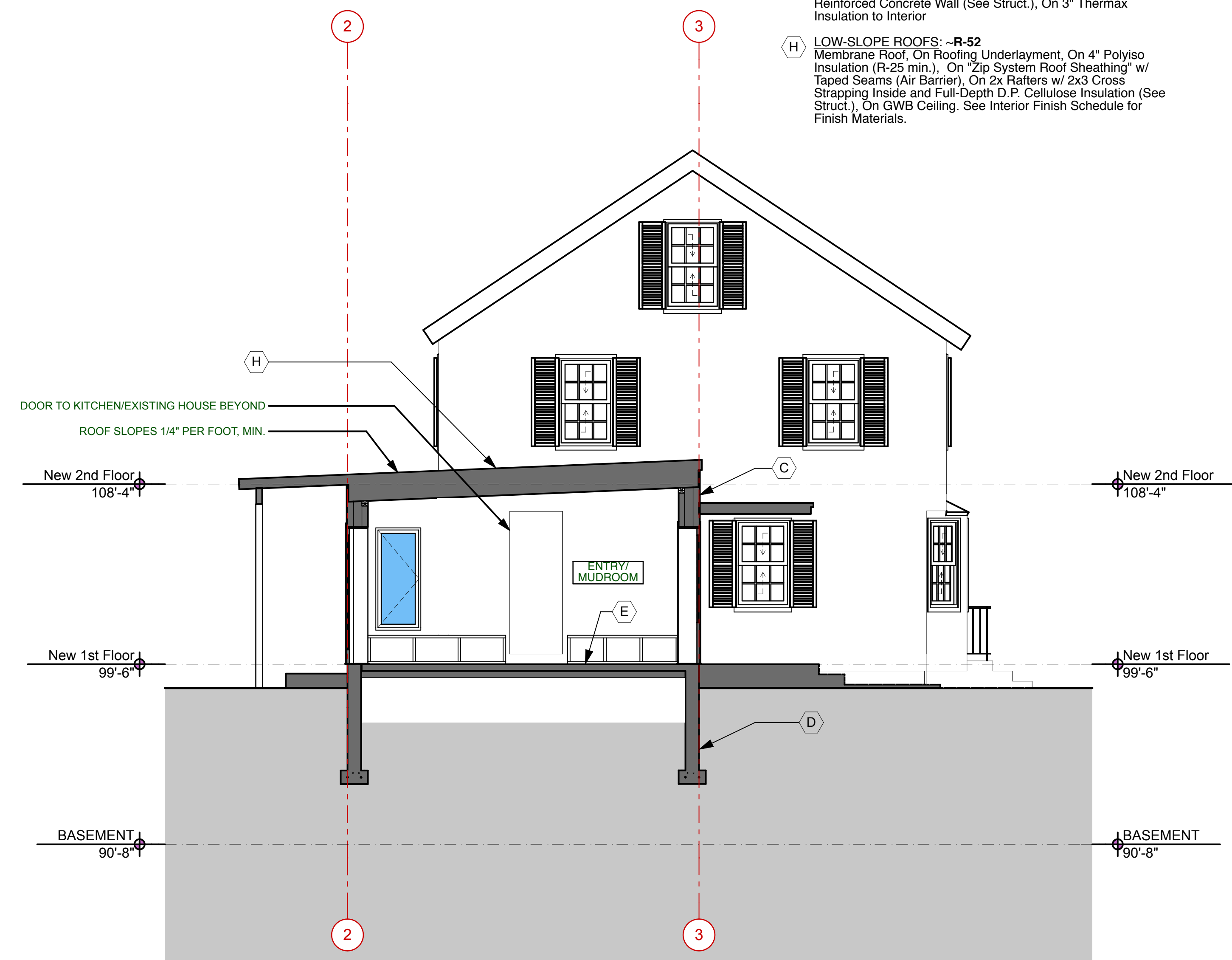
2 Section SCALE: 1/4" = 1'-0"
