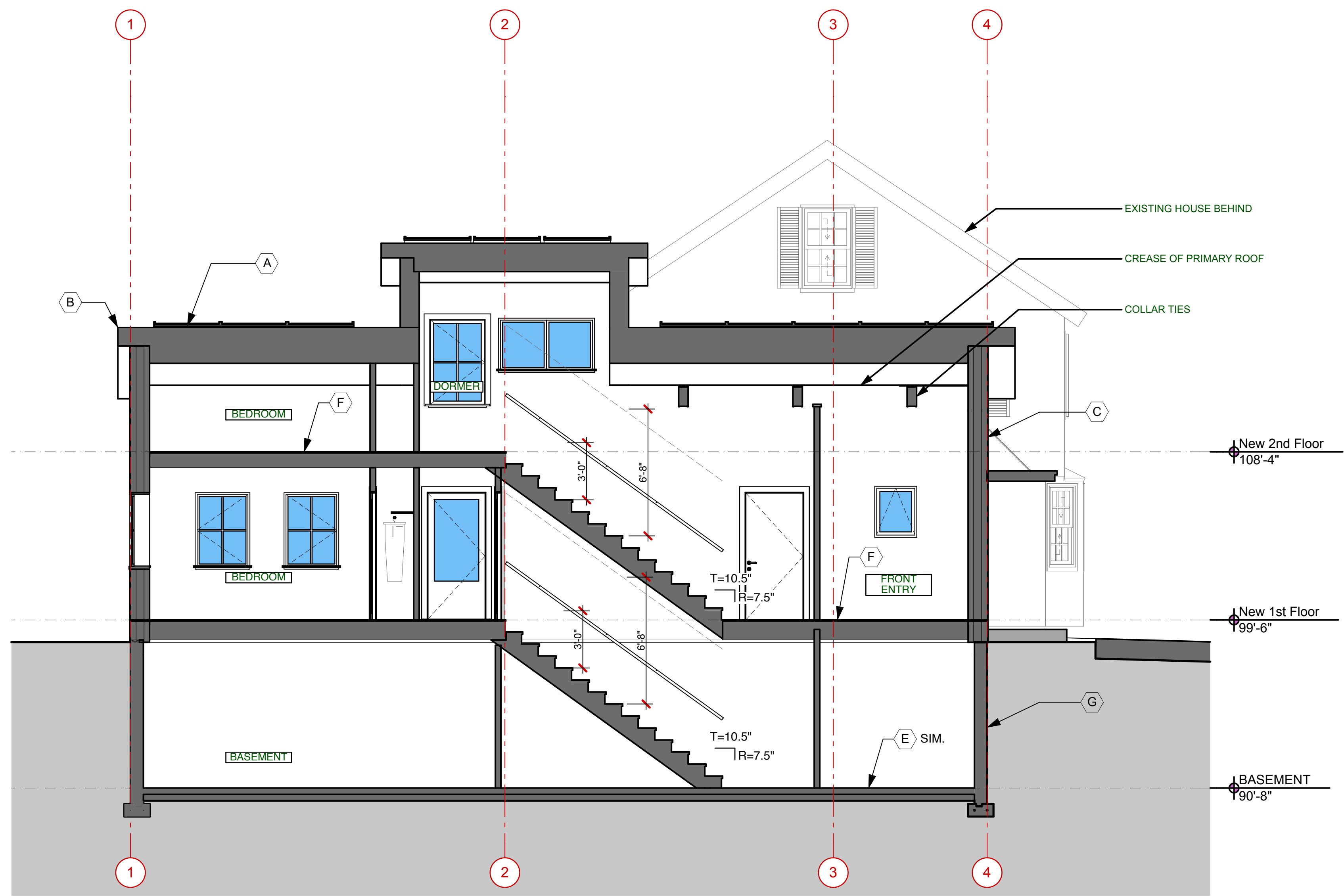
1 Section SCALE: 1/4" = 1'-0"
