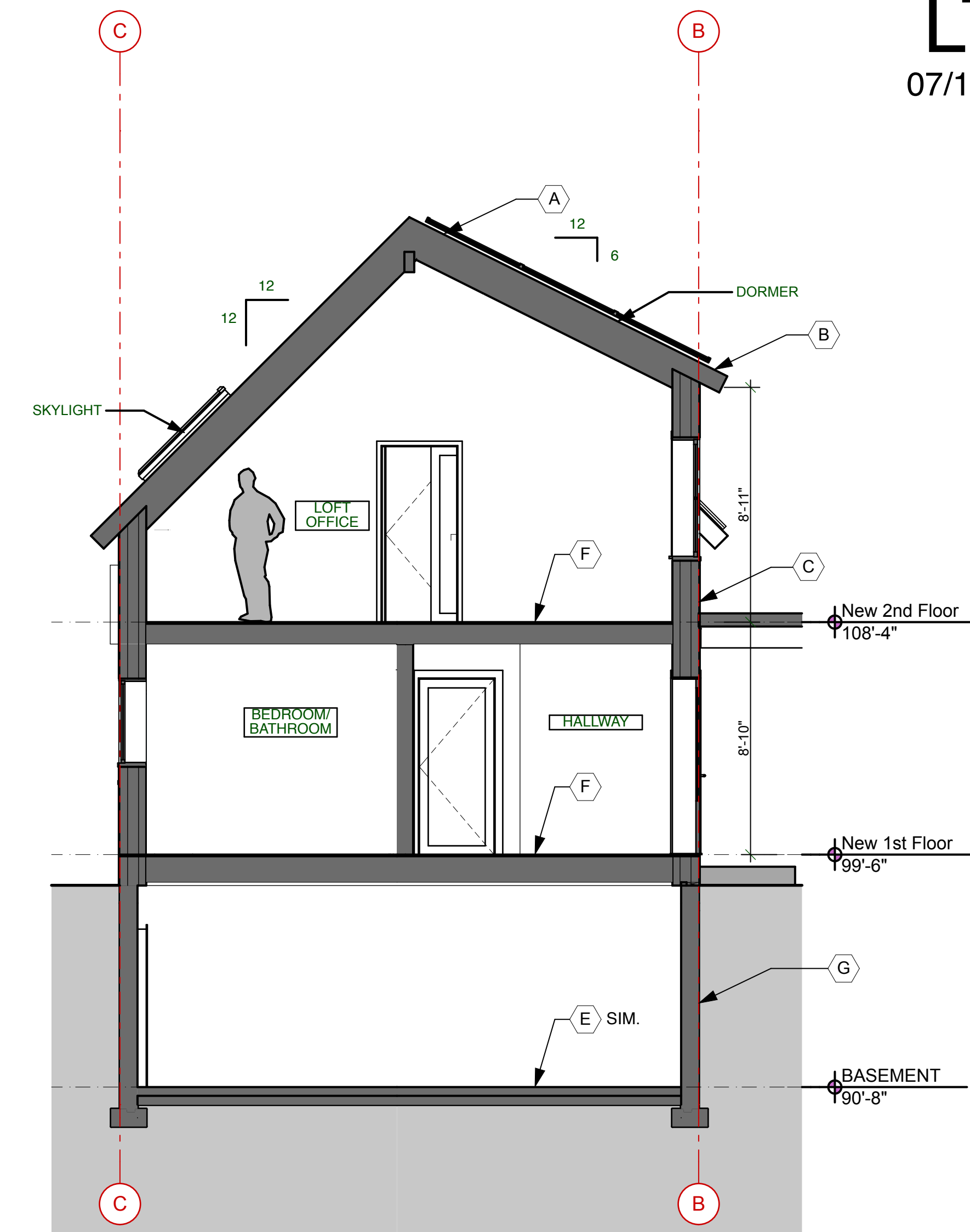
3 Section SCALE: 1/4" = 1'-0"
