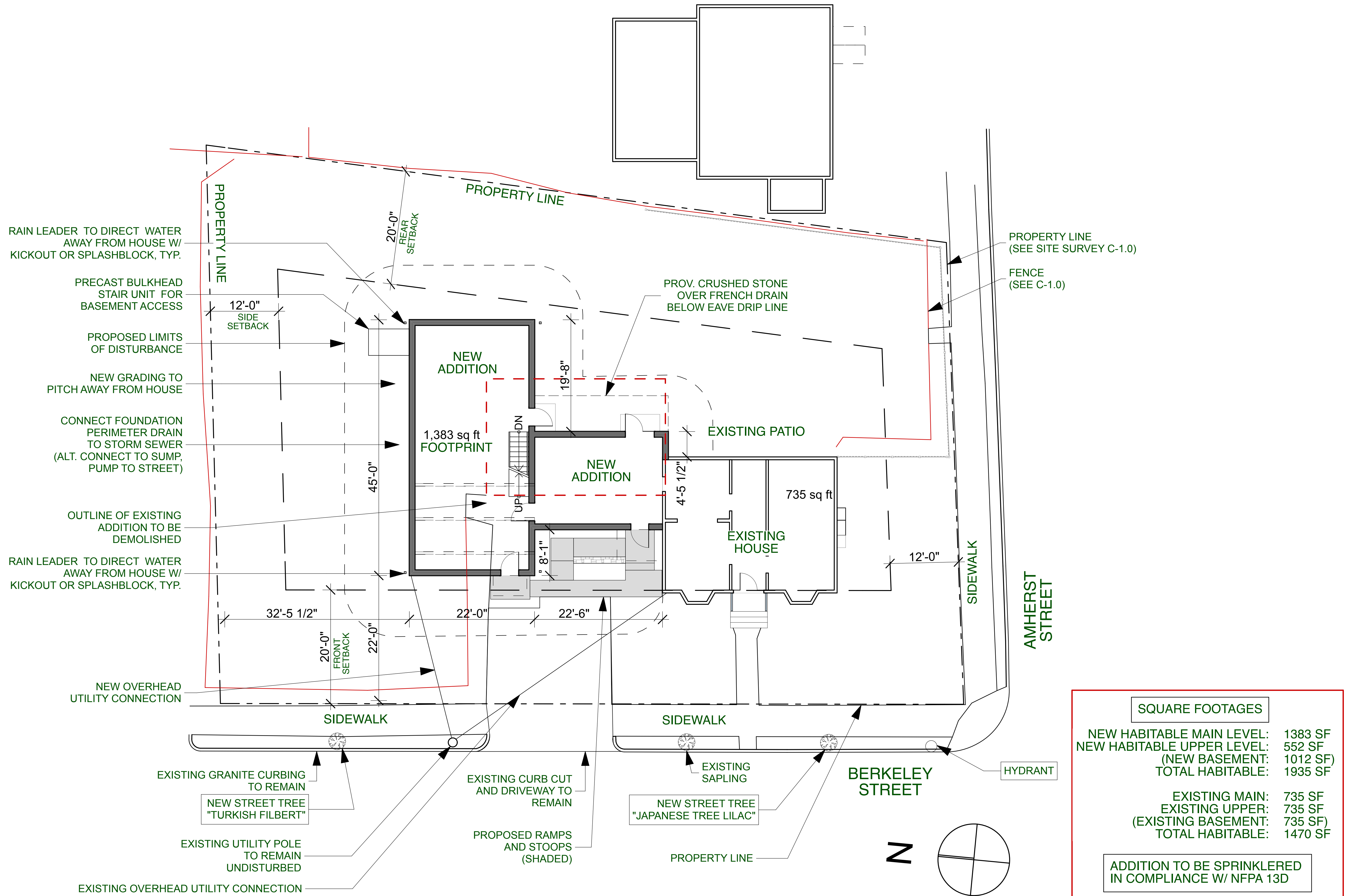
1 SITE PLAN SCALE: 1/8" = 1'-0"
