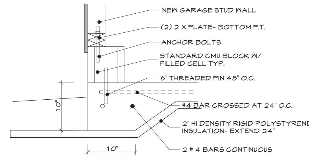
3 Slab Edge SCALE: 1" = 1'-0"
