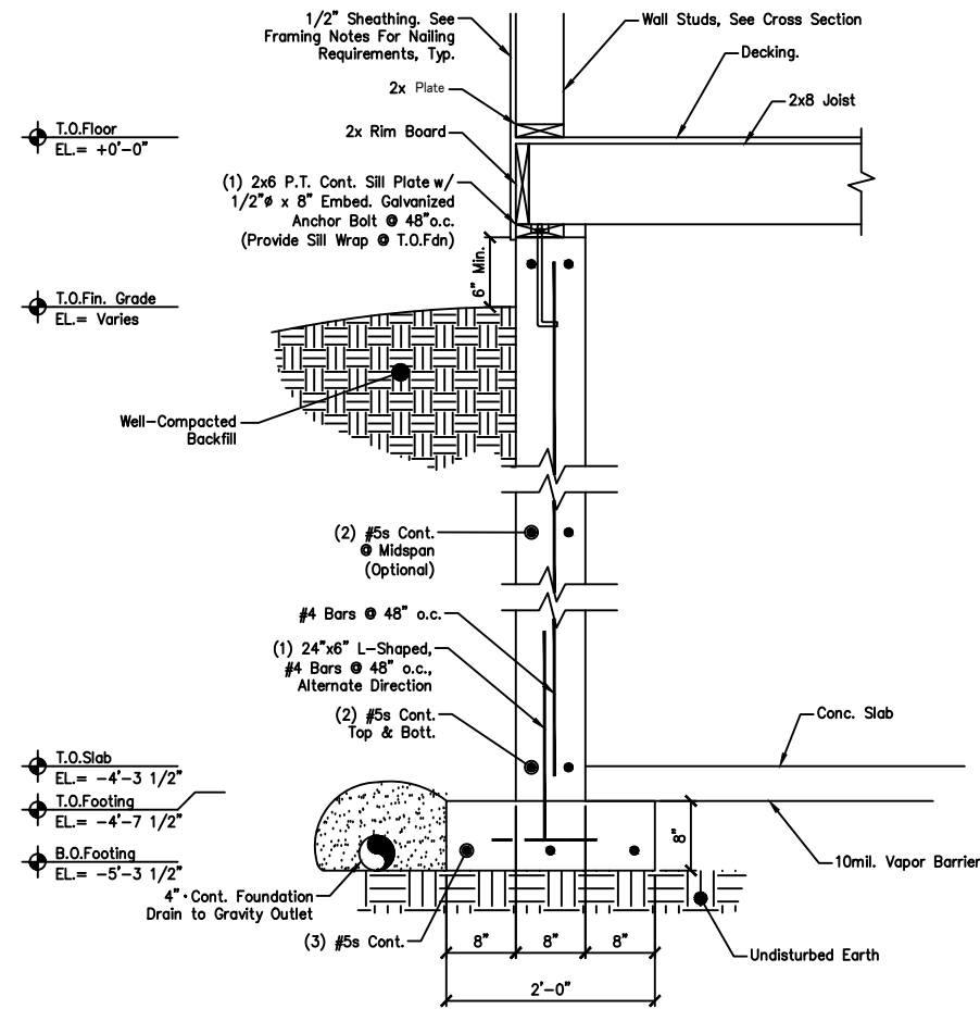
SECTION 1 Scale: 1/2" = 1'-0"
