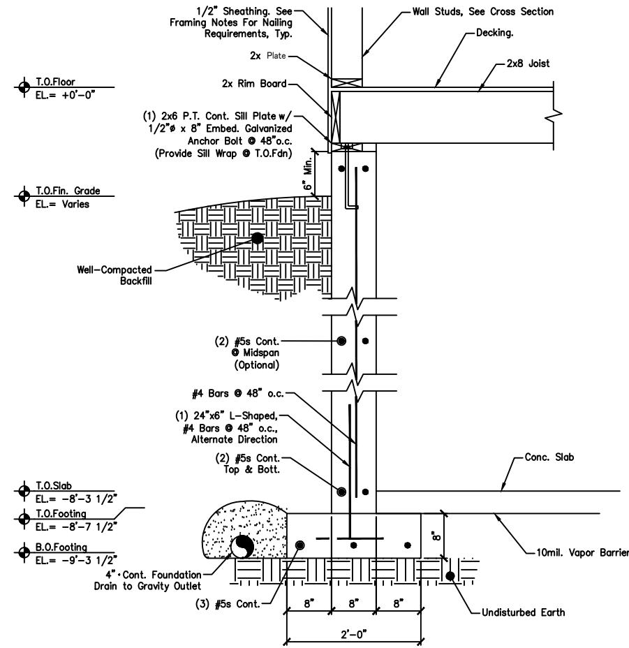
SECTION 2 Scale: 1/2" = 1'-0"
