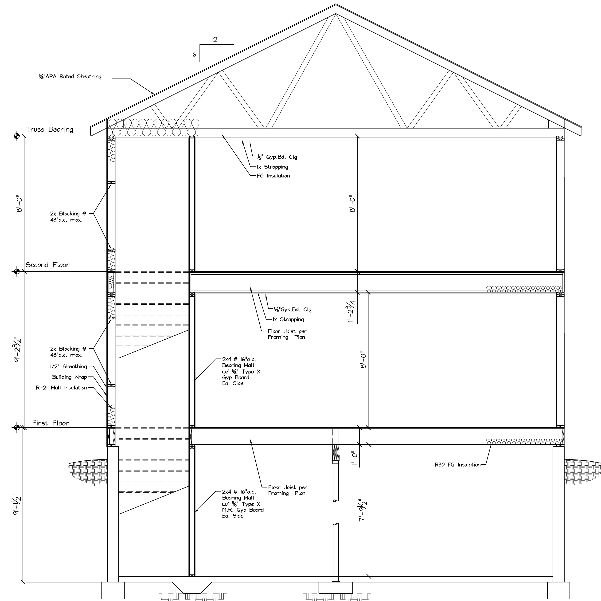
CROSS SECTION B Scale: 3/8" = 1'-0"
