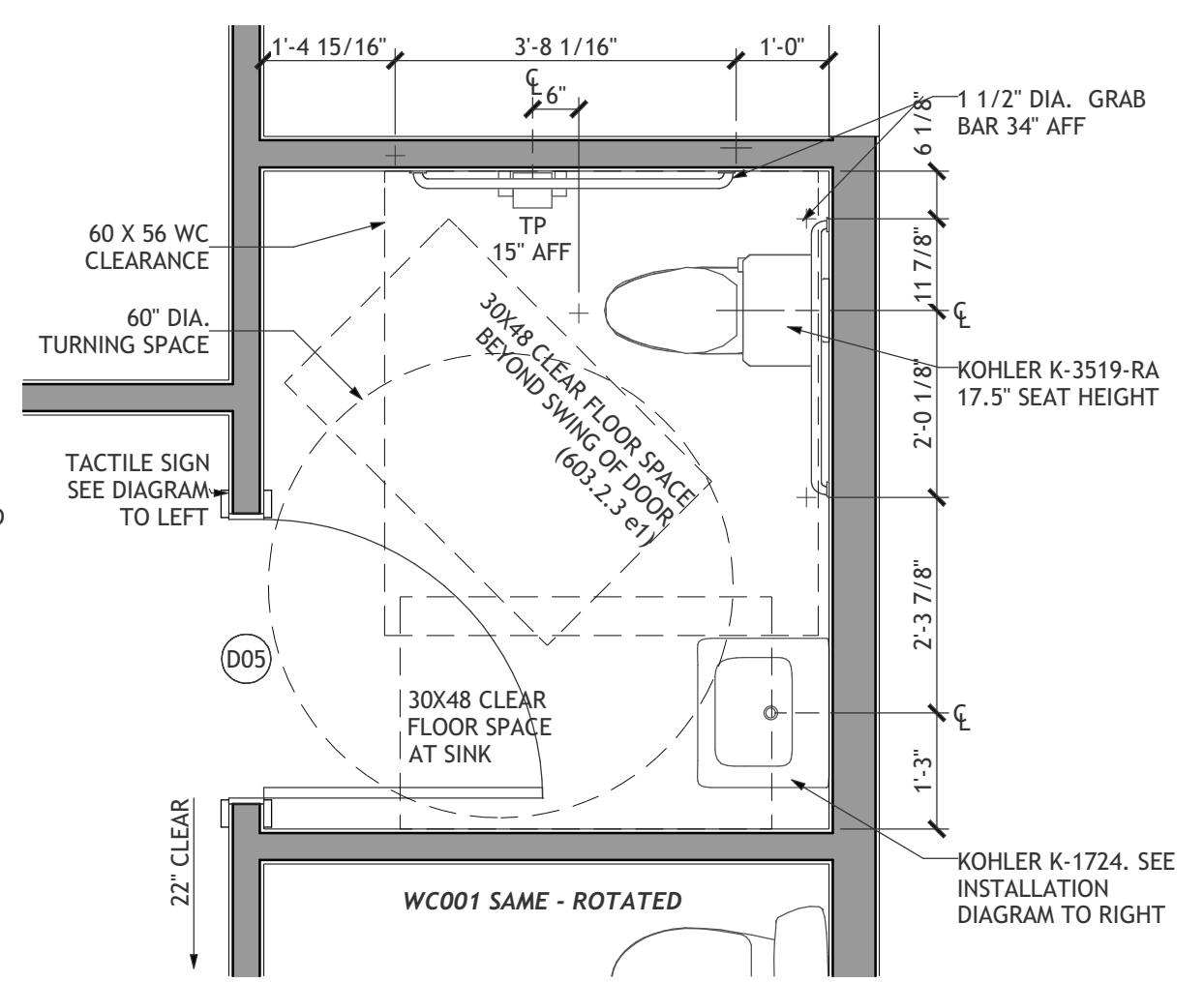
4 : WC Signage : no scale 3 : Enlarged WC101 Plan : 1/2 in = 1 ft 2 : Knee / Toe Clearance
