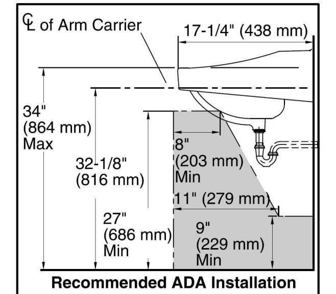
4 : WC Signage : no scale 3 : Enlarged WC101 Plan : 1/2 in = 1 ft 2 : Knee / Toe Clearance
