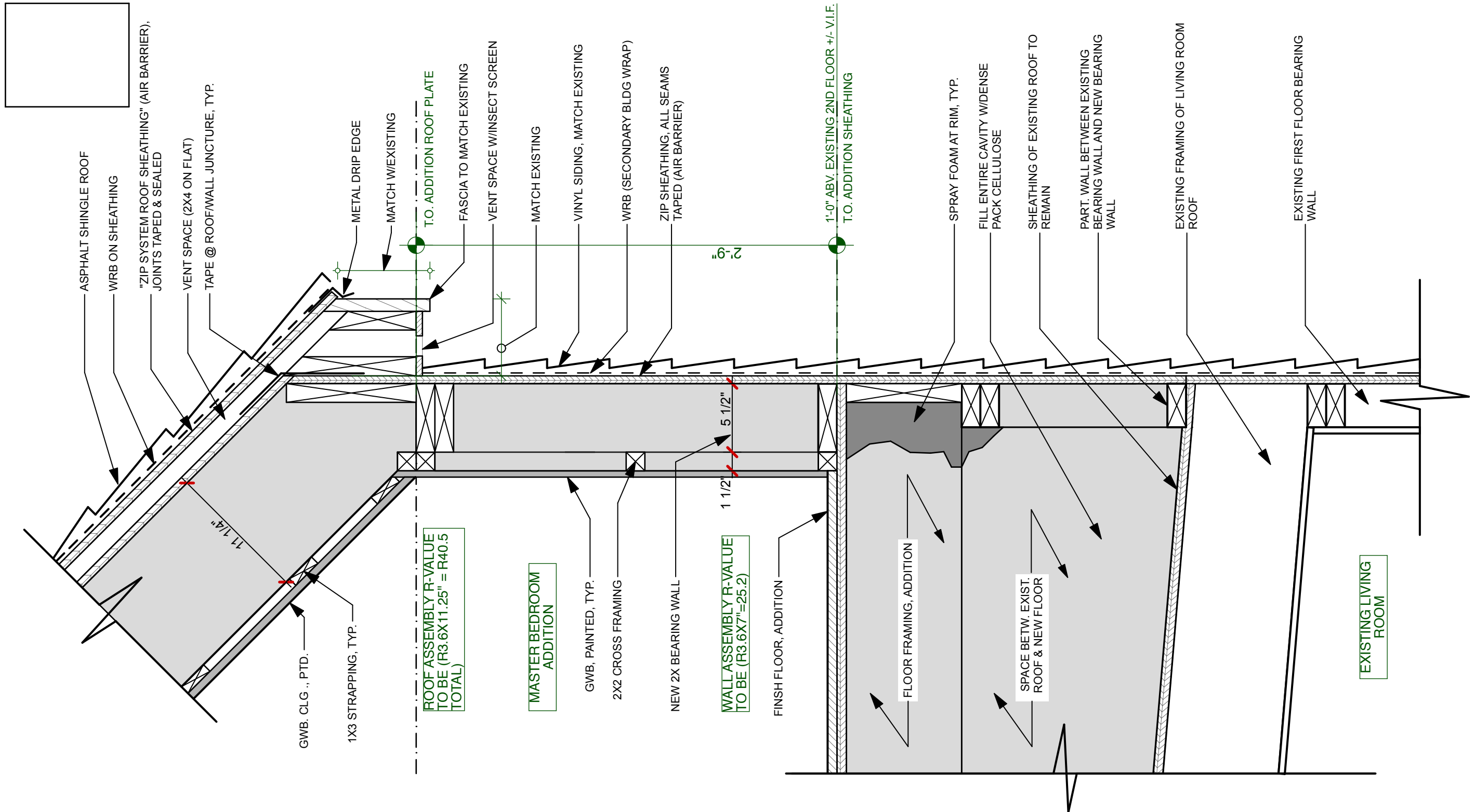
1 Wall Section SCALE: 1 1/2" = 1'-0"
