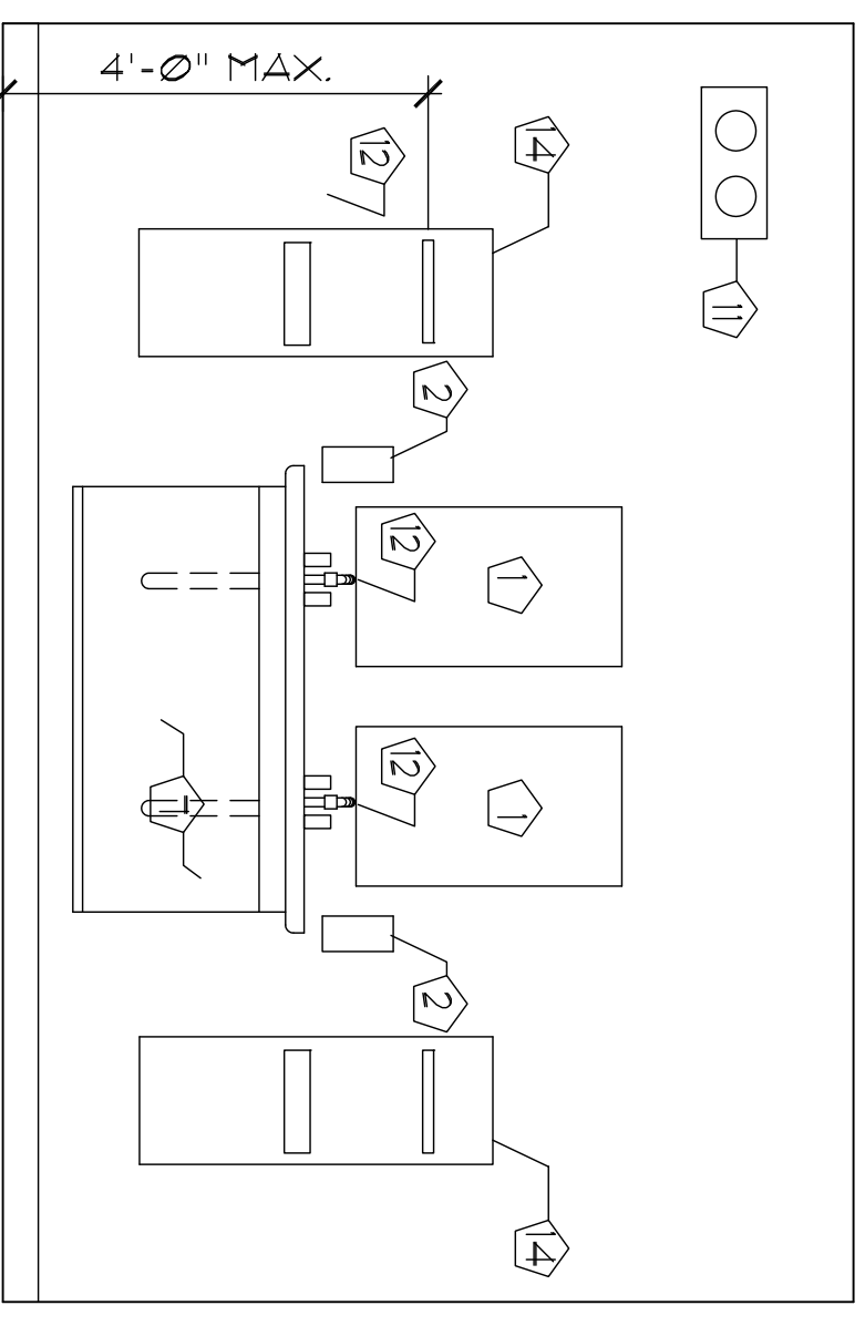
D LAV 109 - ELEVATION SCALE: 1/2" = 1'-0"
