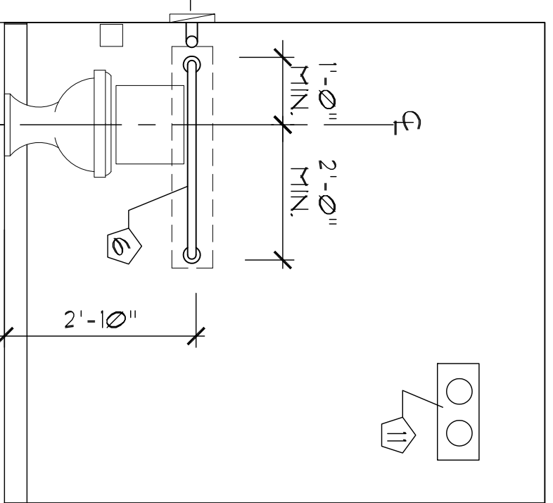
B TLT 104 - ELEVATION SCALE: 1/2" = 1'-0"
