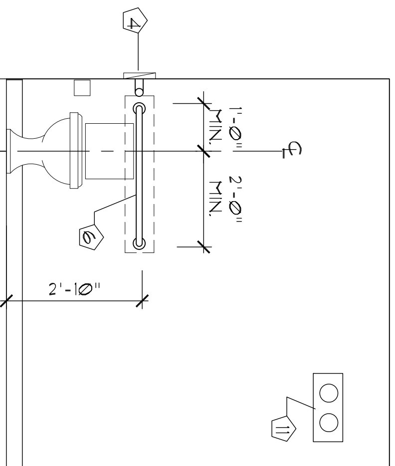
B TLT 104 - ELEVATION SCALE: 1/2" = 1'-0"
