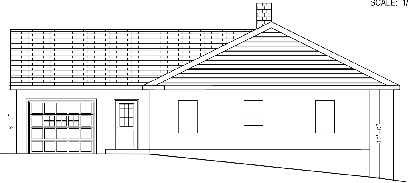
EXISTING FRONT ELEVATION SCALE: 1/8" = 1'-0"
