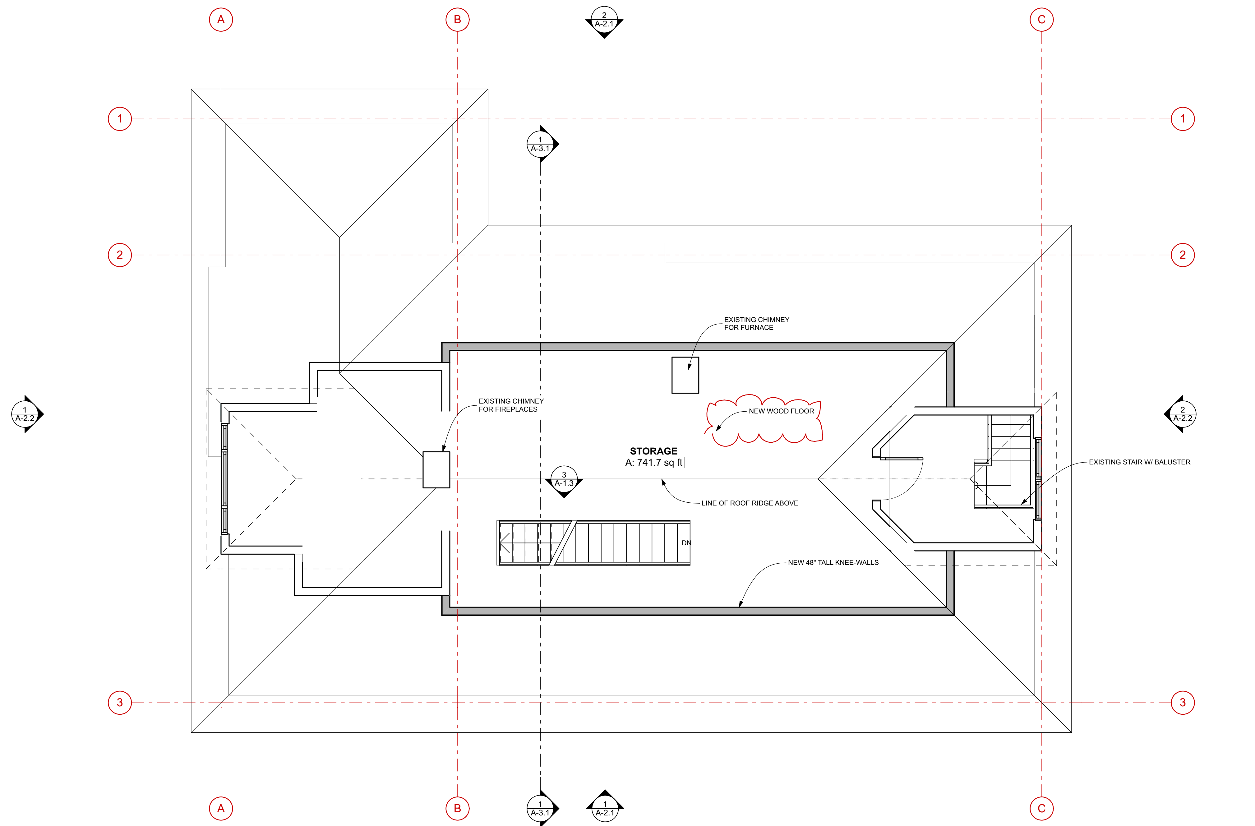
1 ATTIC SCALE: 1/4" = 1'-0"
