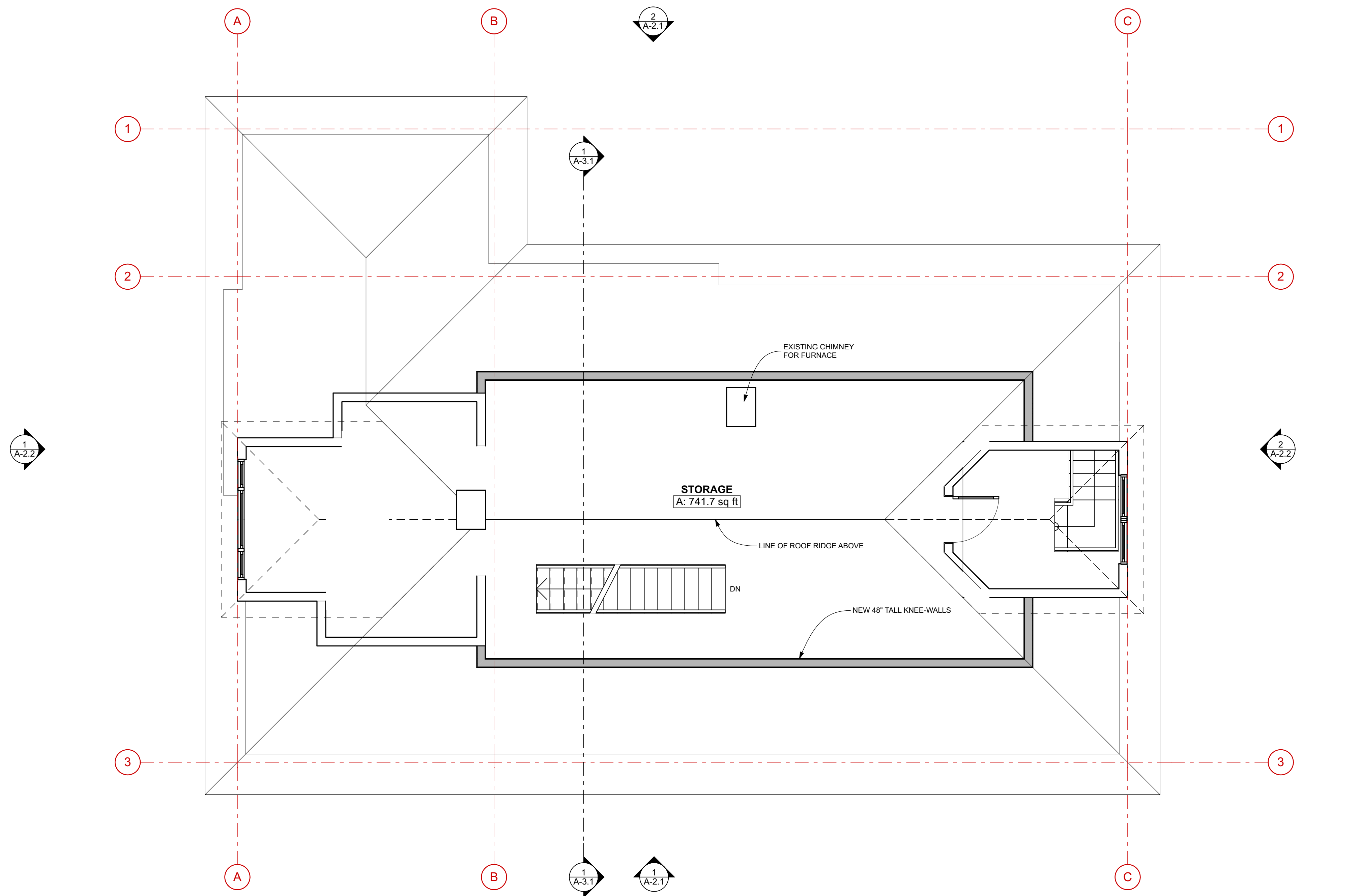
1 ATTIC SCALE: 1/4" = 1'-0"
