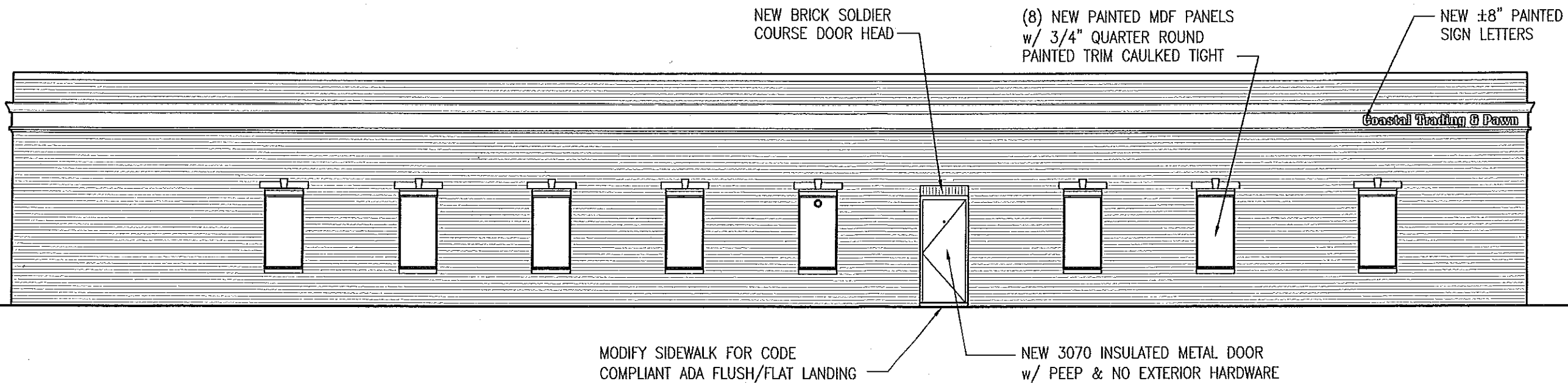
BELMONT ST. ELEVATION SCALE: 1/8" = 1'-0"
