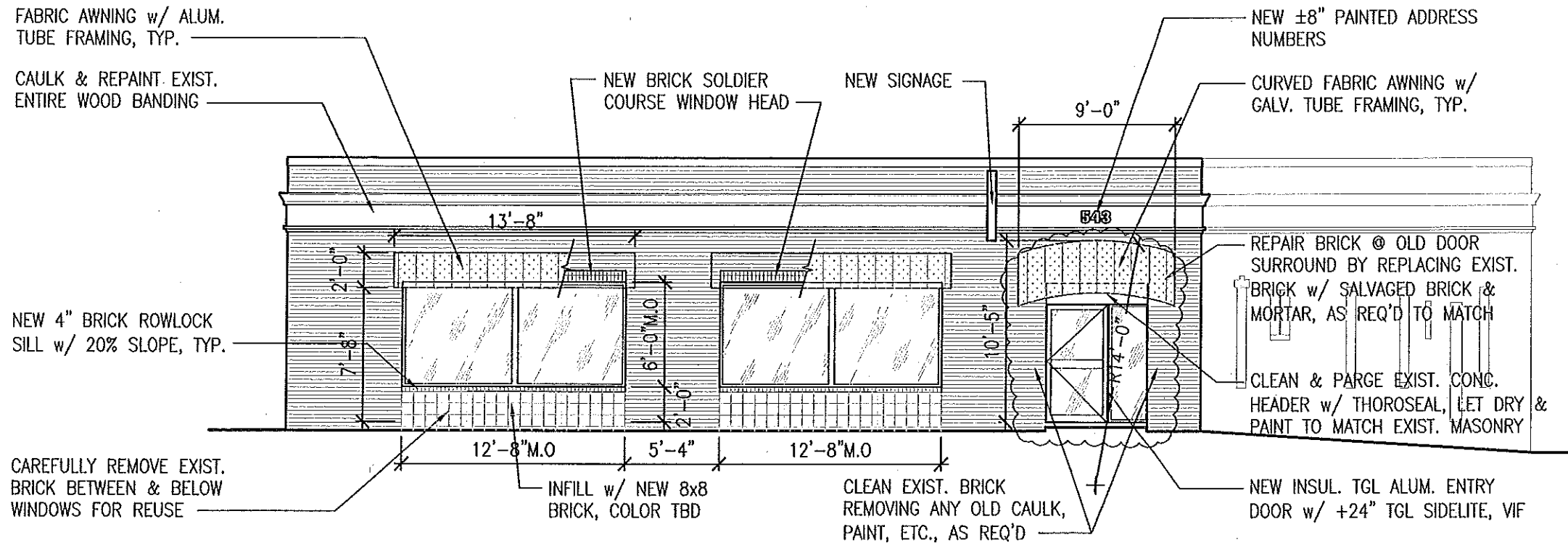
FOREST AVE. ELEVATION SCALE: 1/8" = 1'-0"
