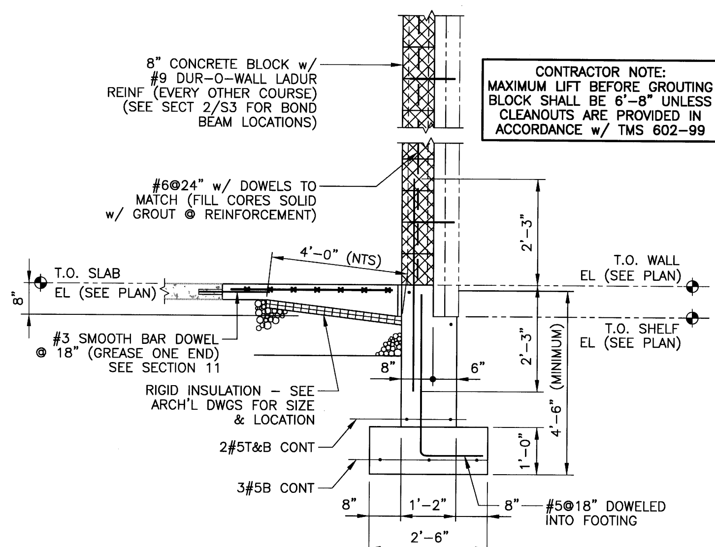
7 SECTION S1 SCALE: 1/2"=1'-0"
