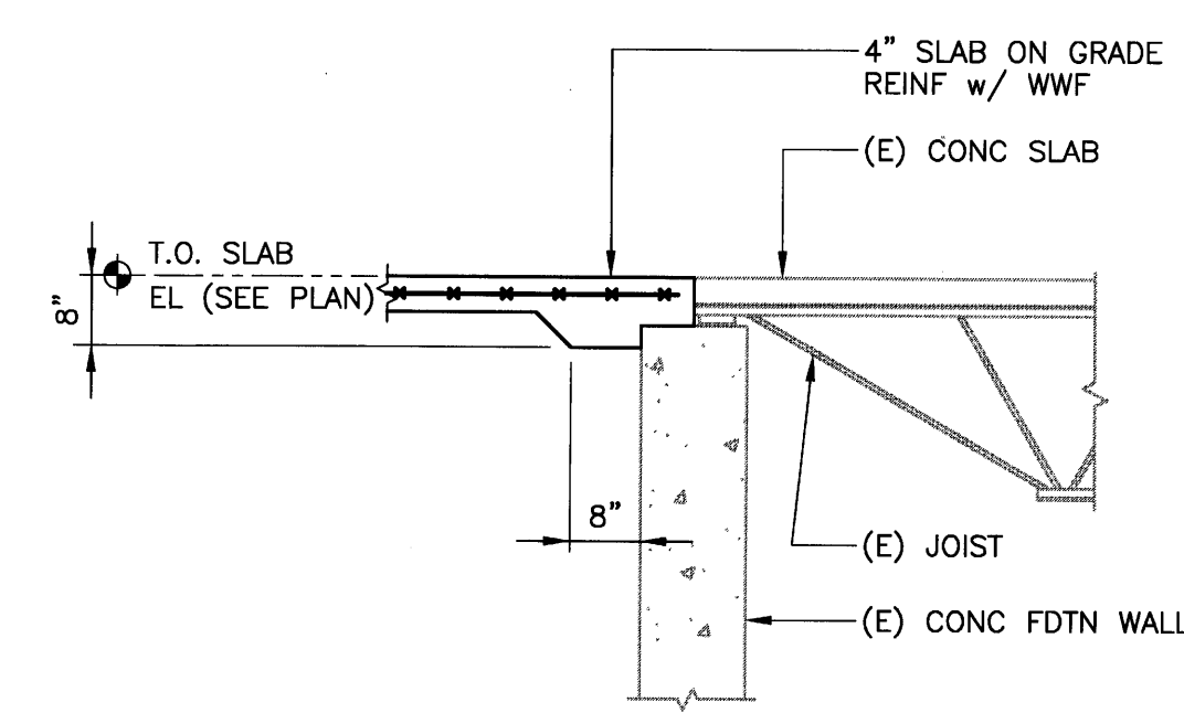
9 SECTION S1 SCALE: 1/2"=1'-0"
