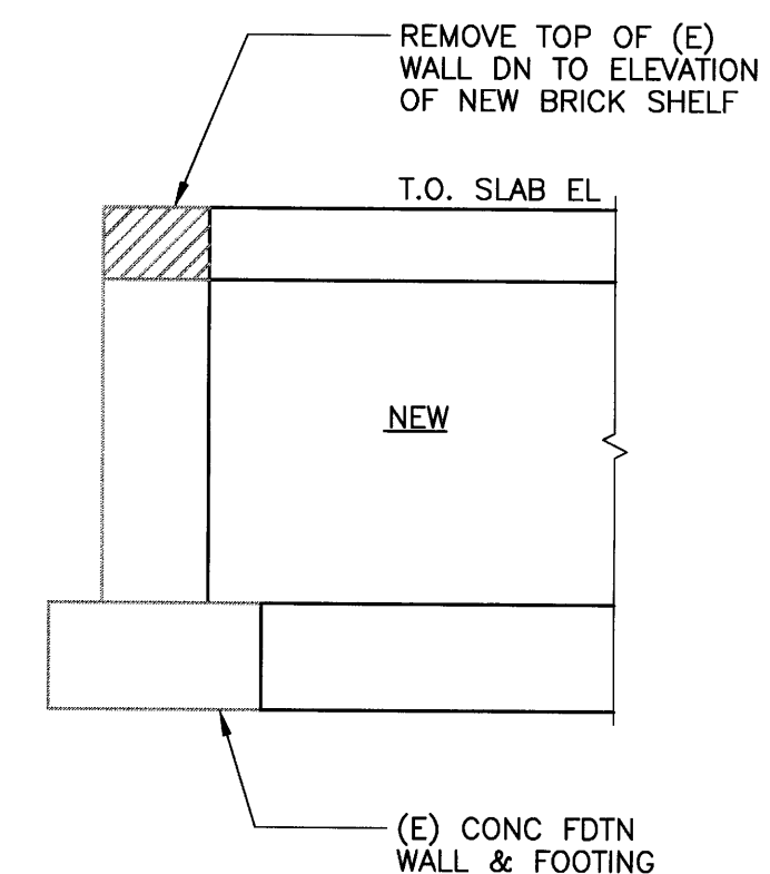
13 SECTION S1 SCALE: 1/2"=1'-0"
