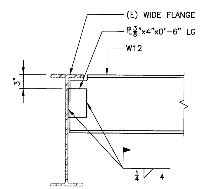
9 SECTION S1 SCALE: 1/2"=1'-0"
