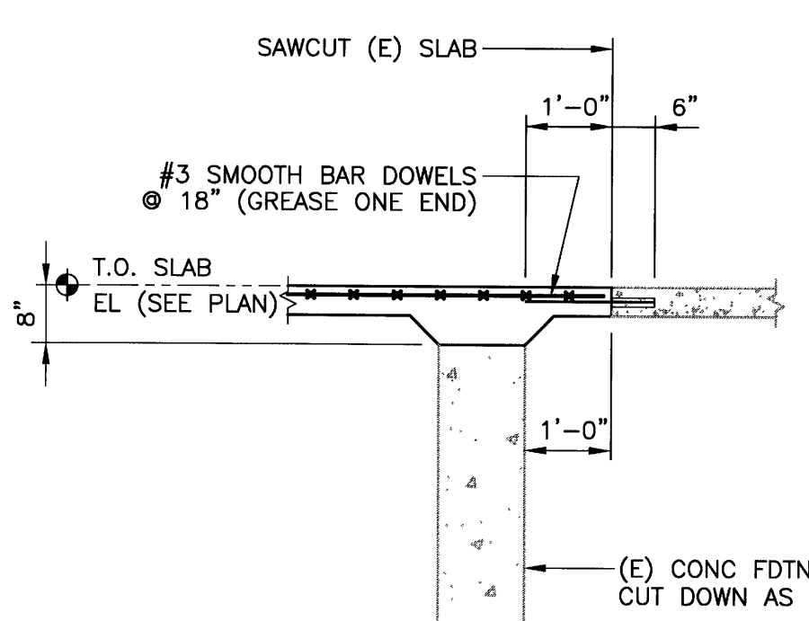
7 SECTION S1 SCALE: 1/2"=1'-0"
