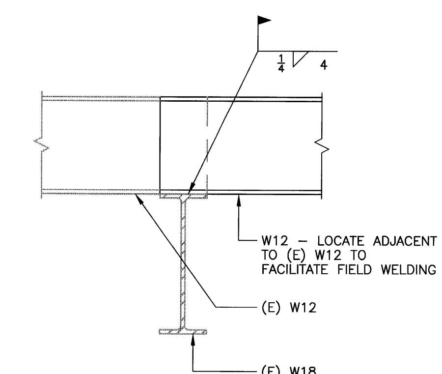
15 SECTION S1 SCALE: 1"=1'-0"
