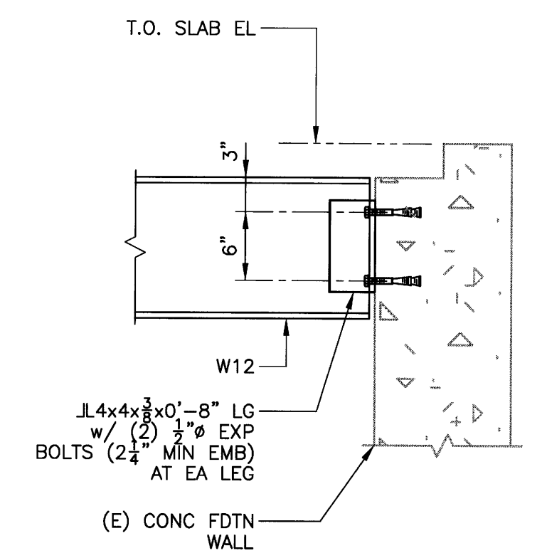
17 SECTION S1 SCALE: 1"=1'-0"
