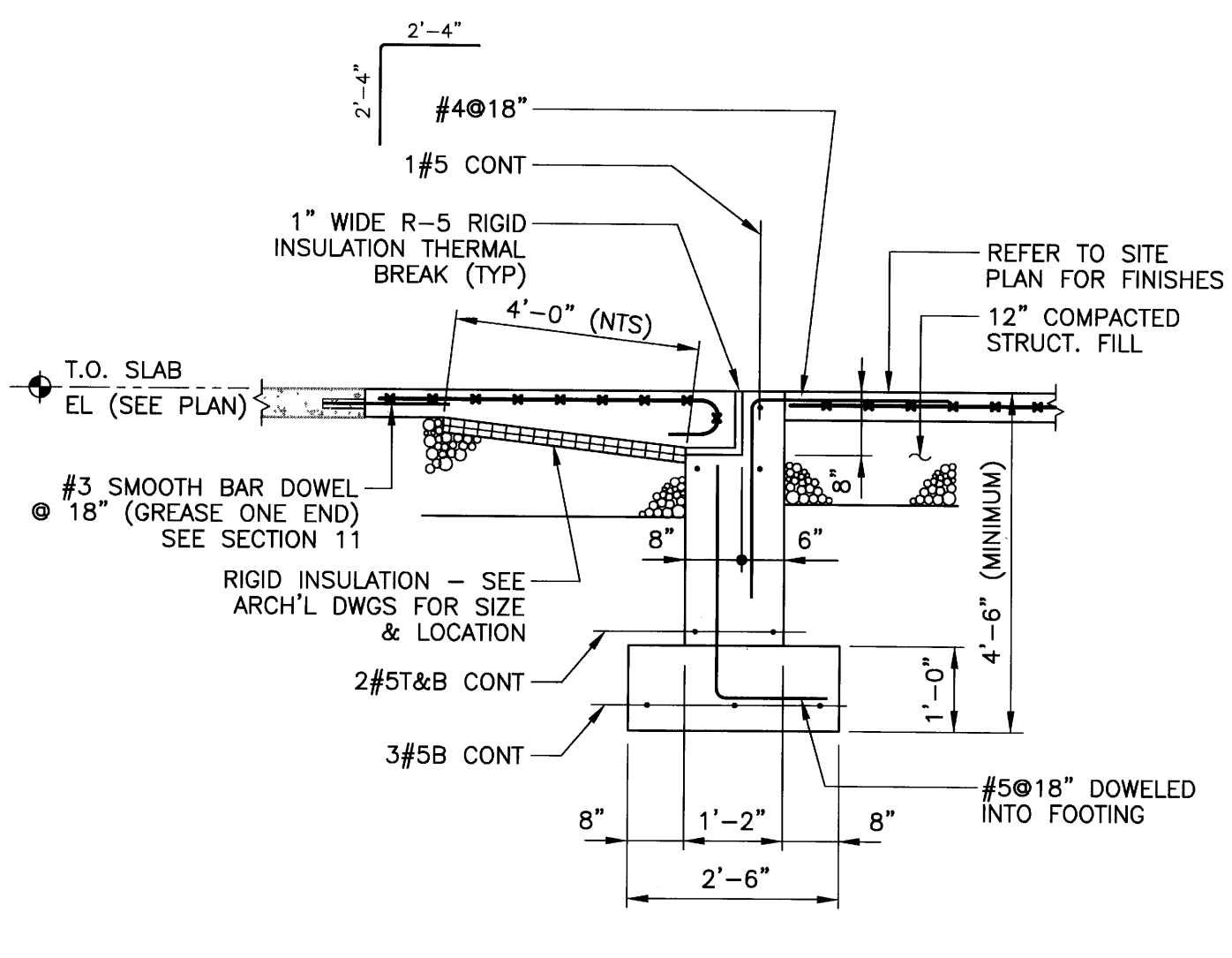
8 SECTION S1 SCALE: 1/2"=1'-0"
