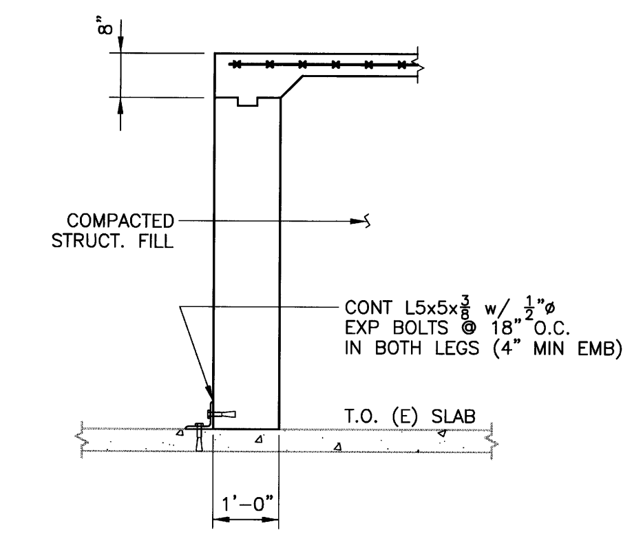
20 SECTION S1 SCALE: 1/2"=1'-0"
