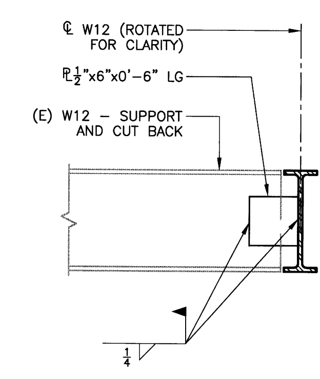
18 SECTION S1 SCALE: 1"=1'-0"
