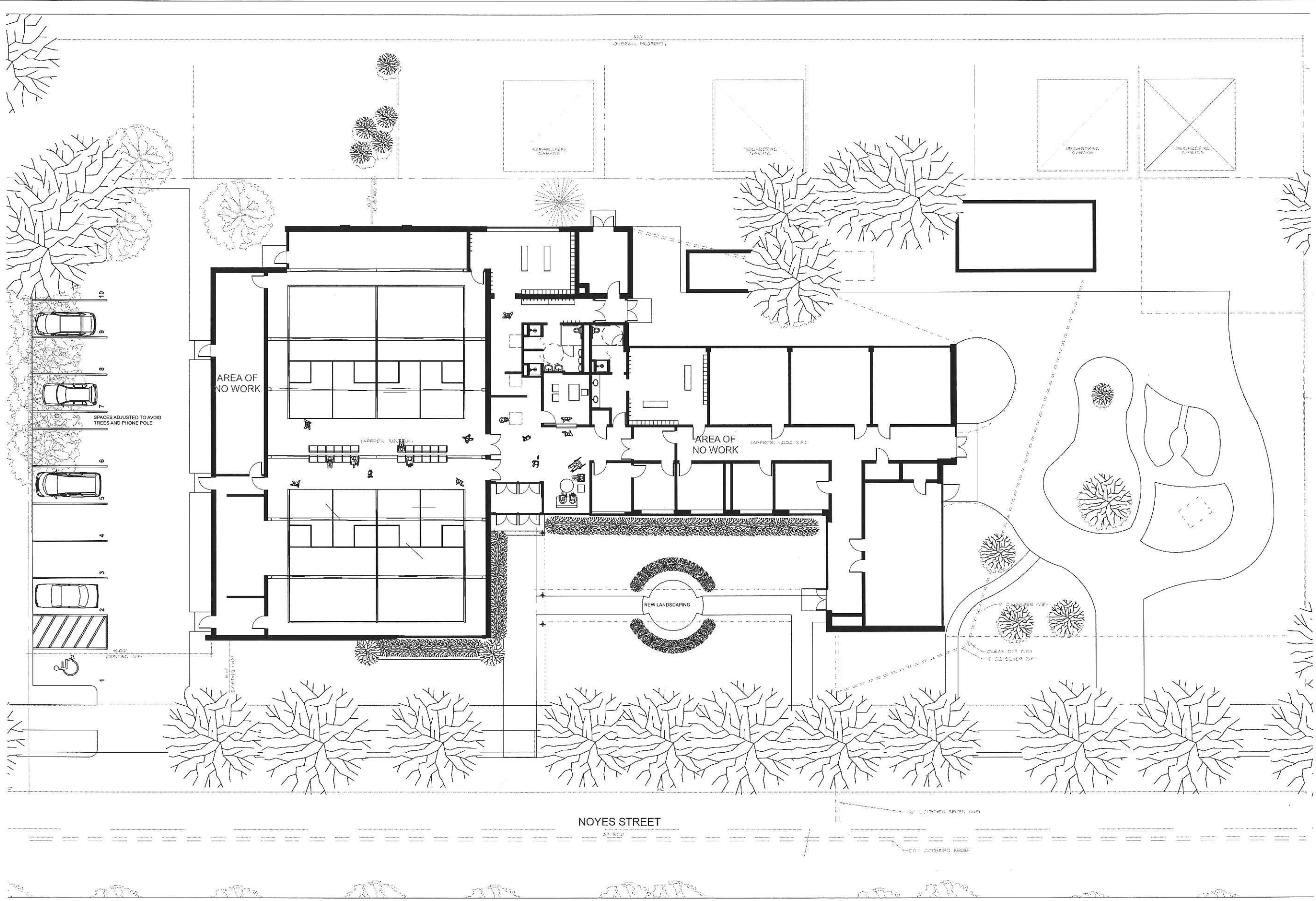
1 SITE PLAN A-1.2 SCALE: 1" = 10'
