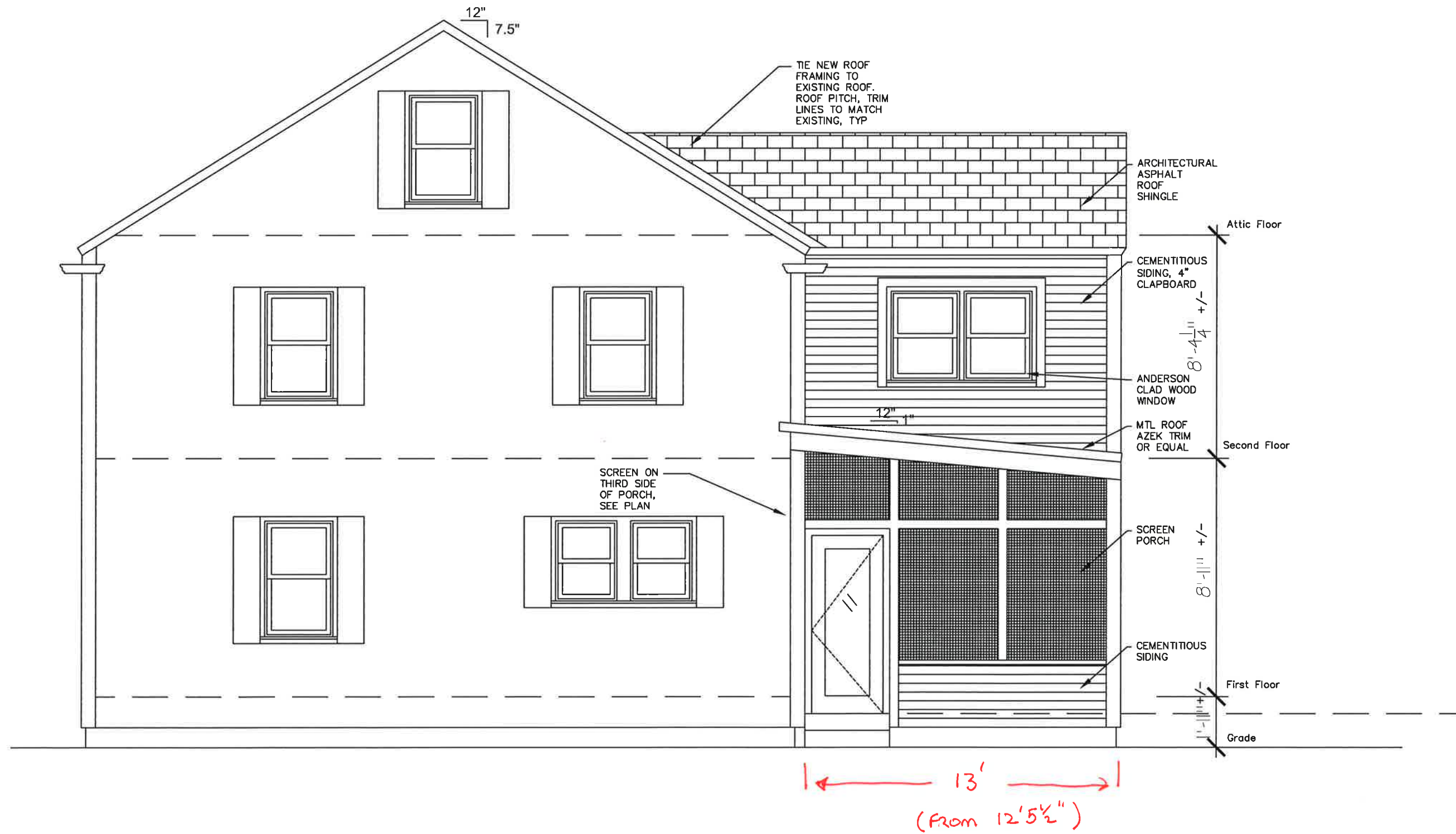
1 ELEVATION SCALE: 1/4" = 1'-0"
