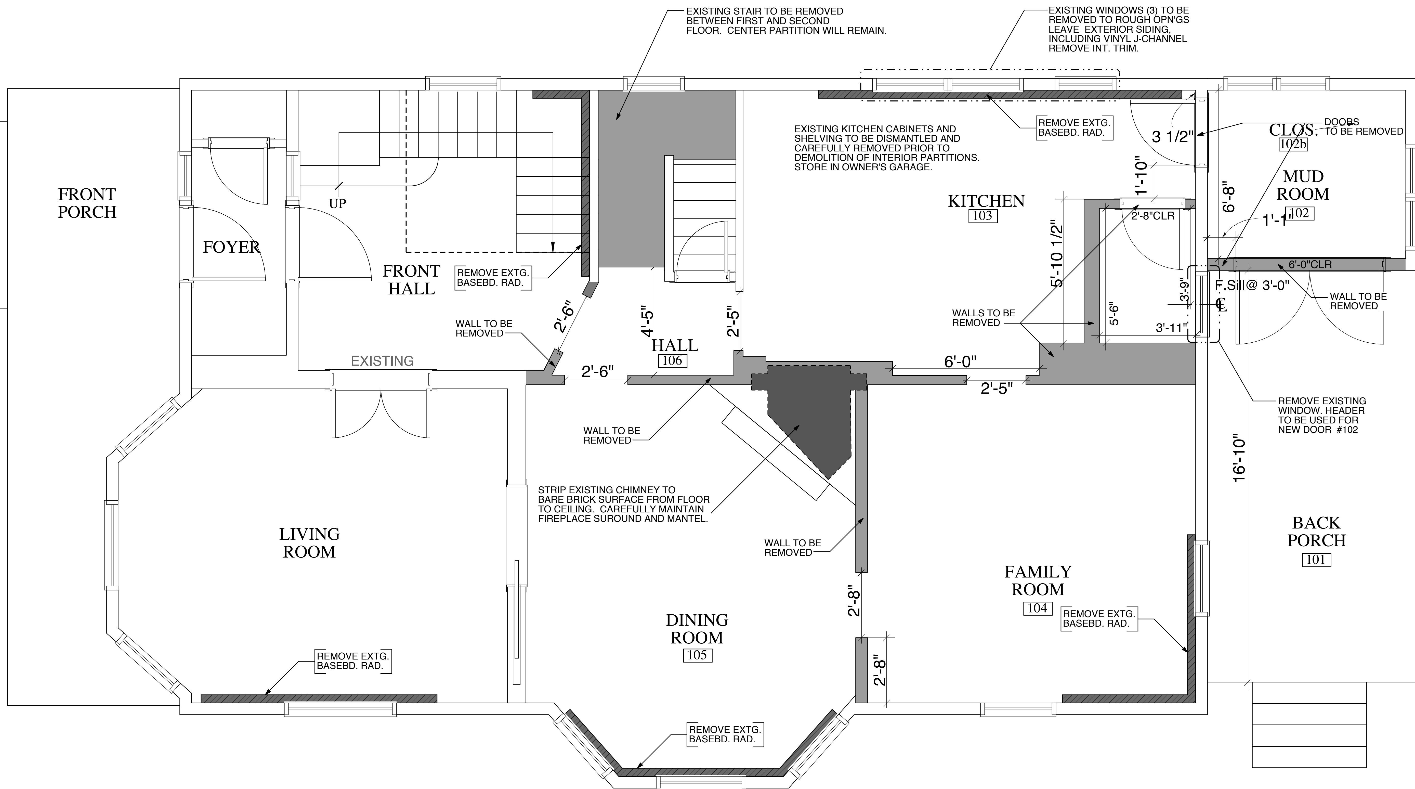
D1.1 DEMOLITION PLAN SCALE: 1/2" = 1'-0"
