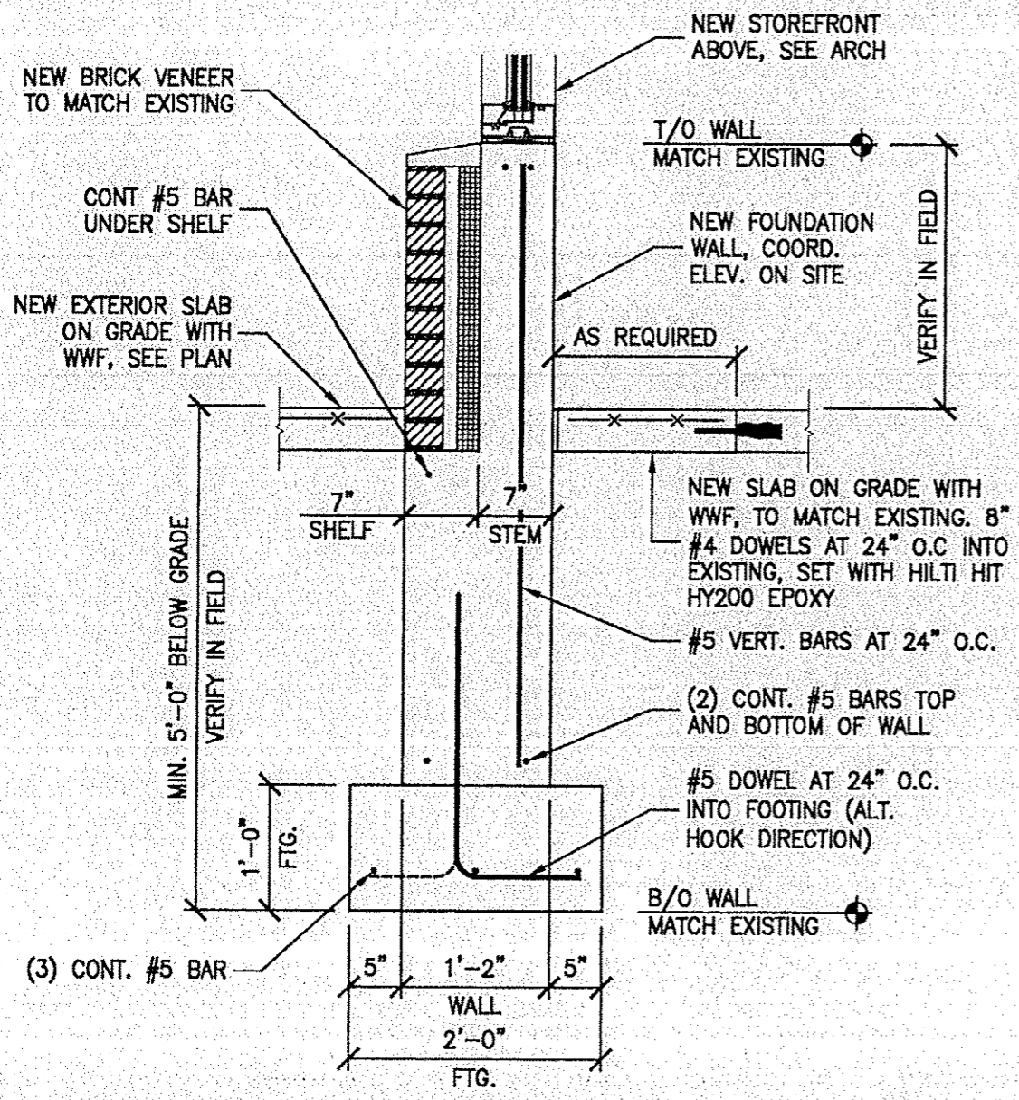
1 SECTION SCALE: 3/4" = 1'-0"
