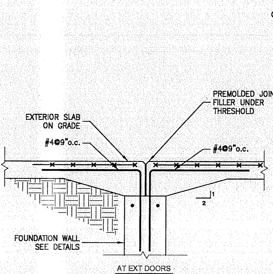
2 TYPICAL OVER POUR DETAILS SCALE: N.T.S.
