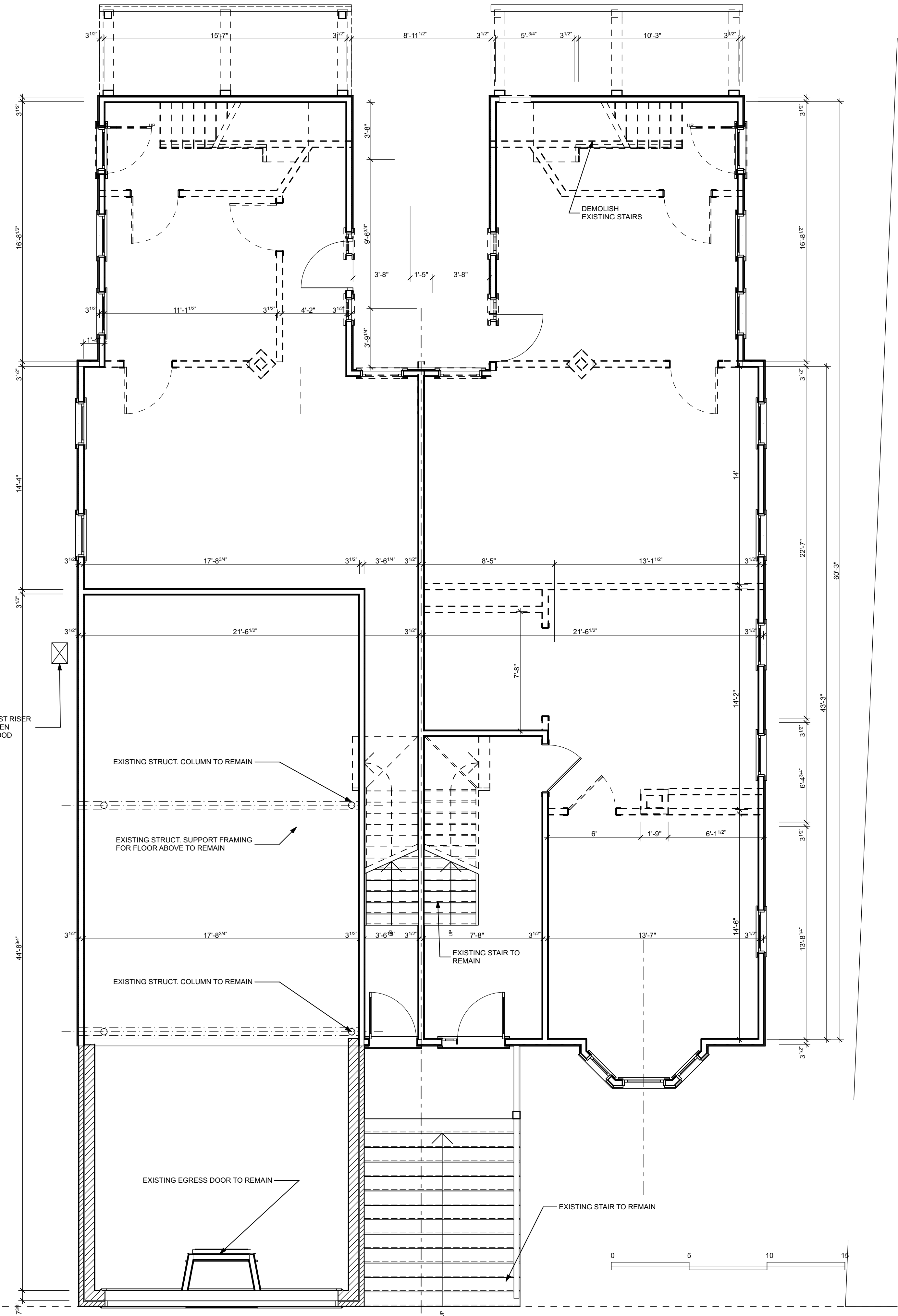
2 D1.1 FIRST FLOOR DEMO SCALE: 1/4" = 1'-0"
