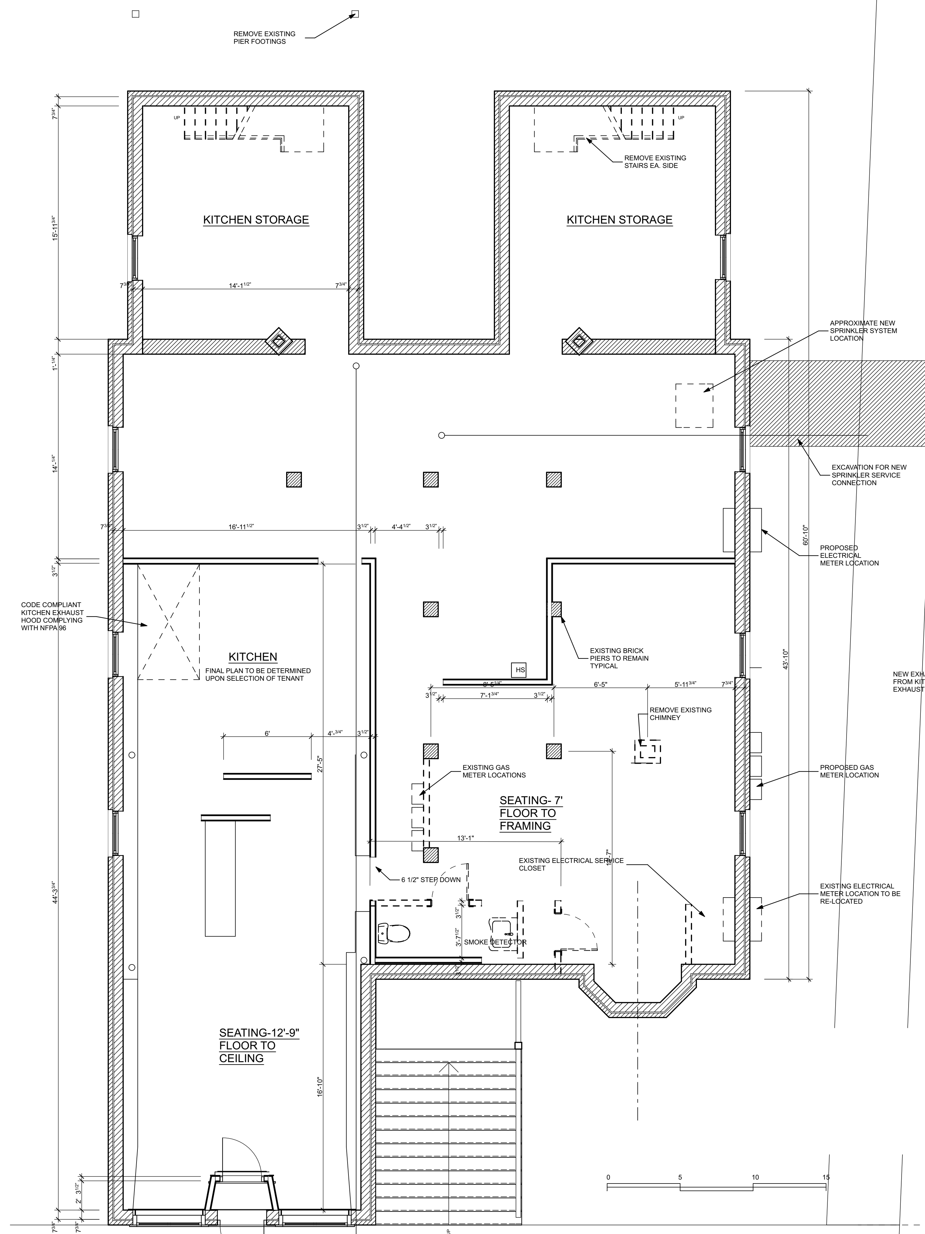
1 D1.1 BASEMENT DEMO PLAN SCALE: 1/4" = 1'-0"
