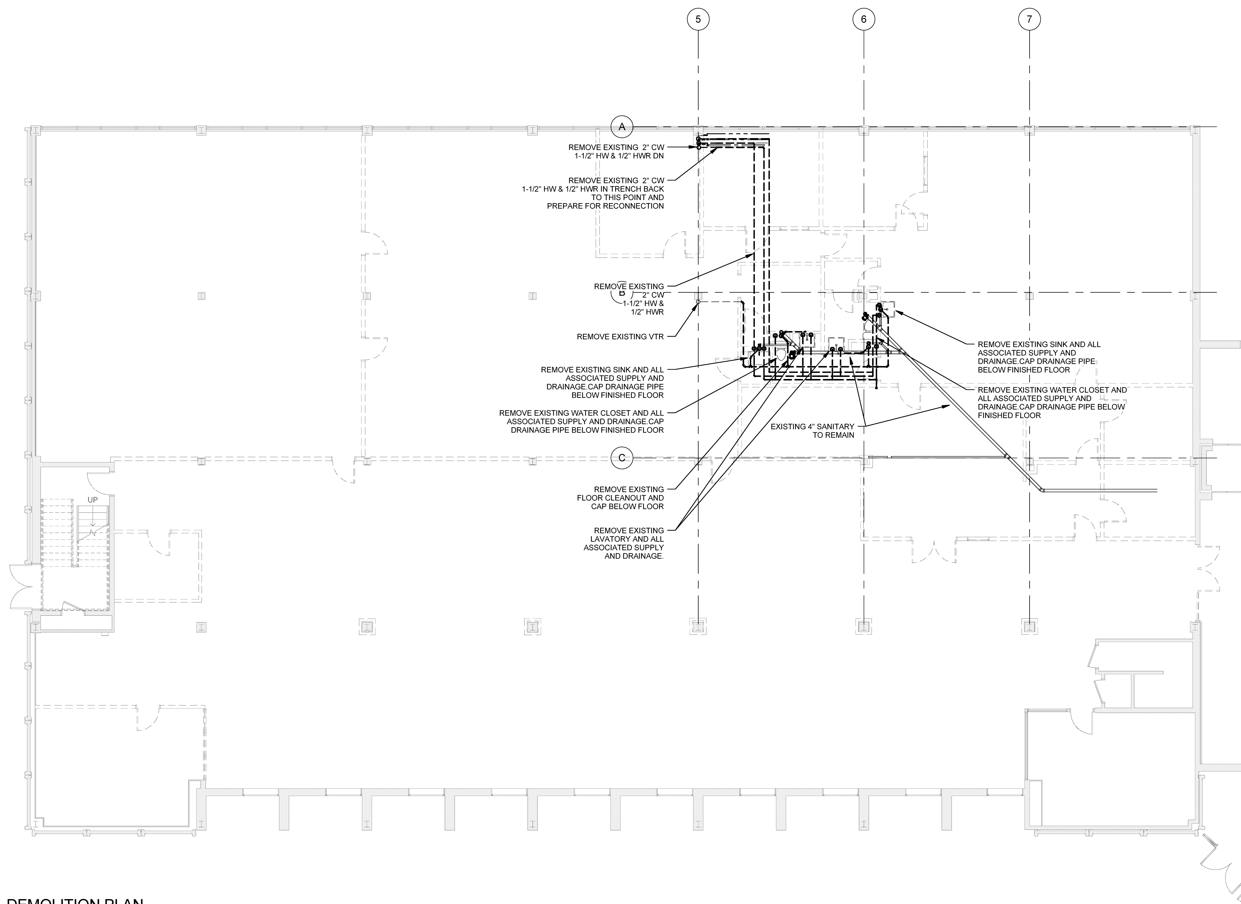
1 DEMOLITION PLAN SCALE: 1/8" = 1'-0"
