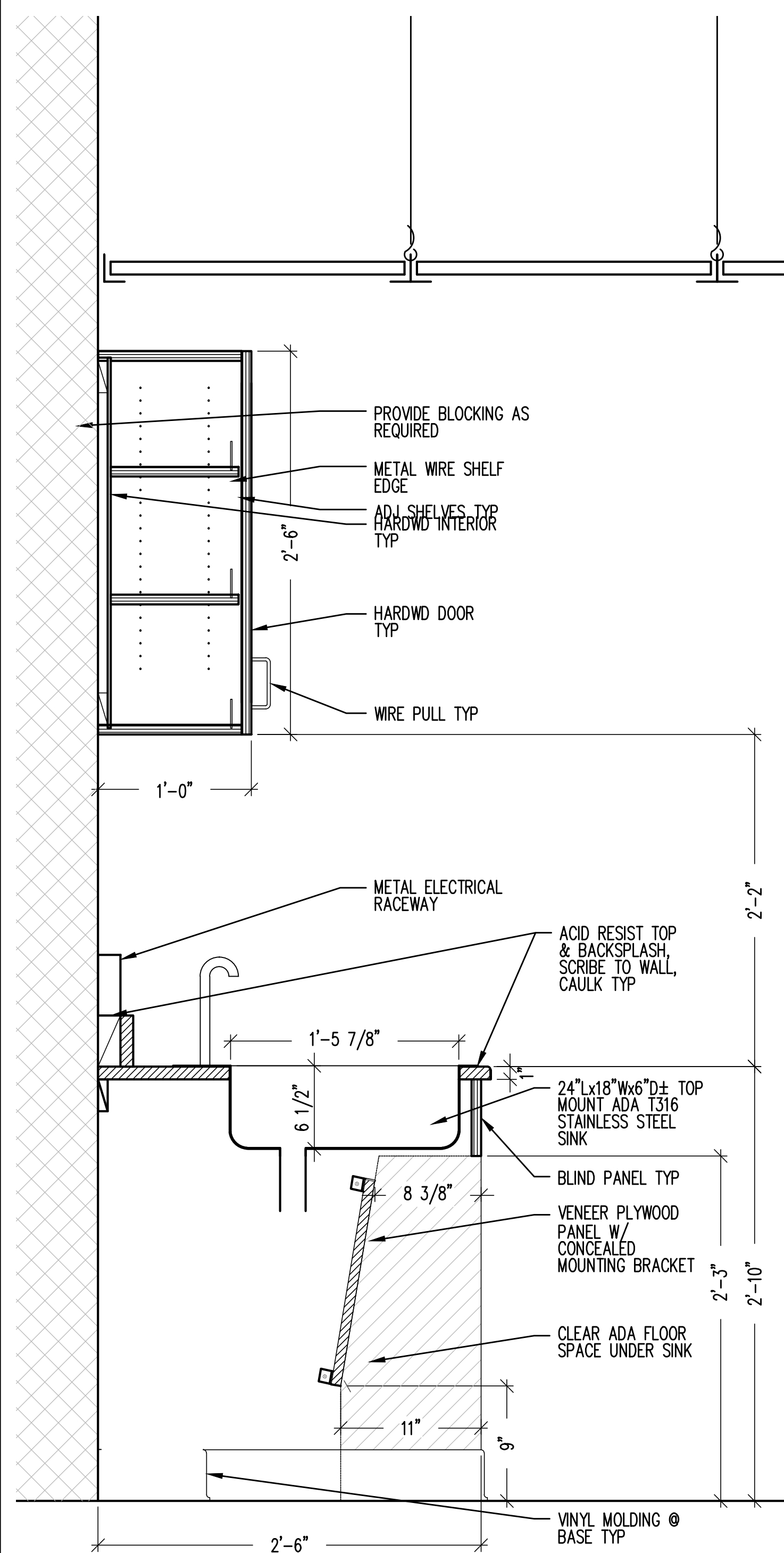
1 SECTION A1.1/A3.1 SCALE: 1-1/2" = 1'-0"
