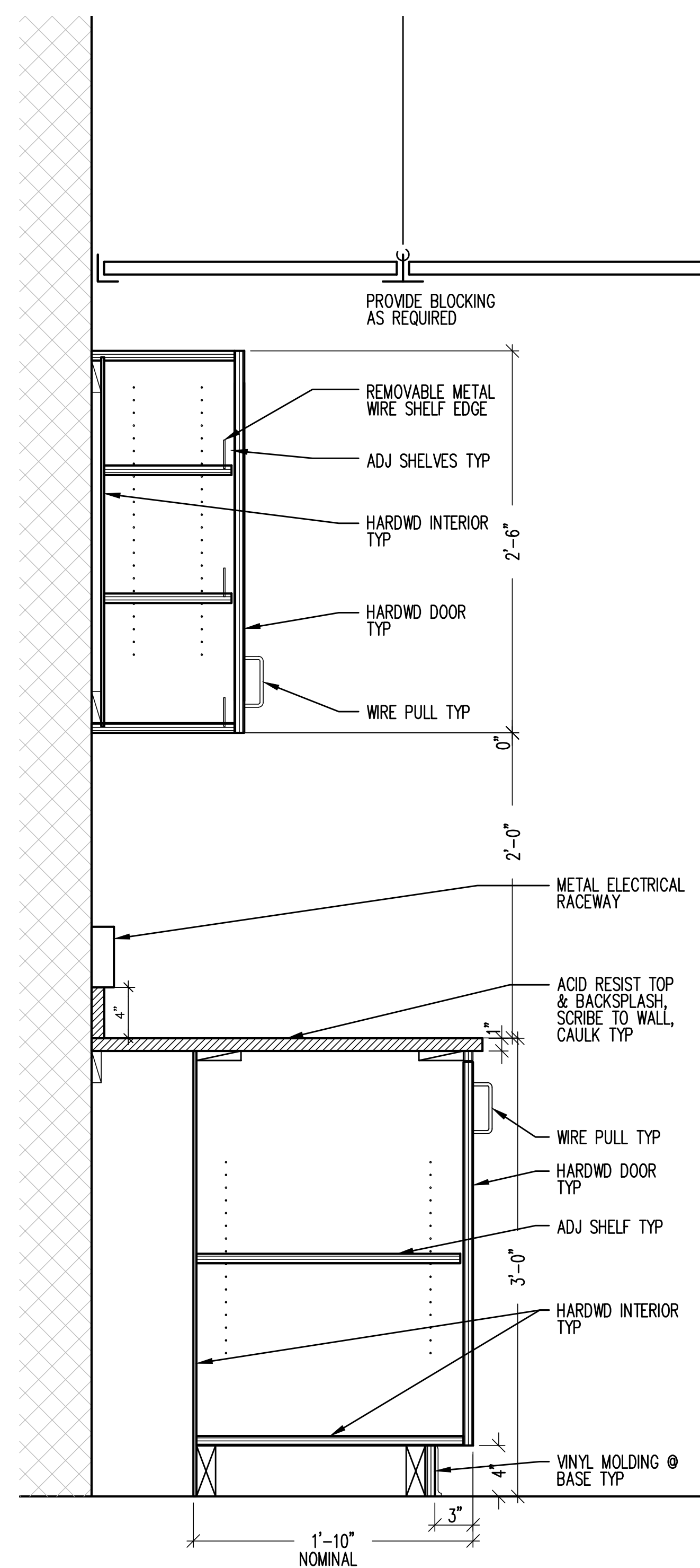
2 SECTION A1.1/A3.1 SCALE: 1-1/2" = 1'-0"
