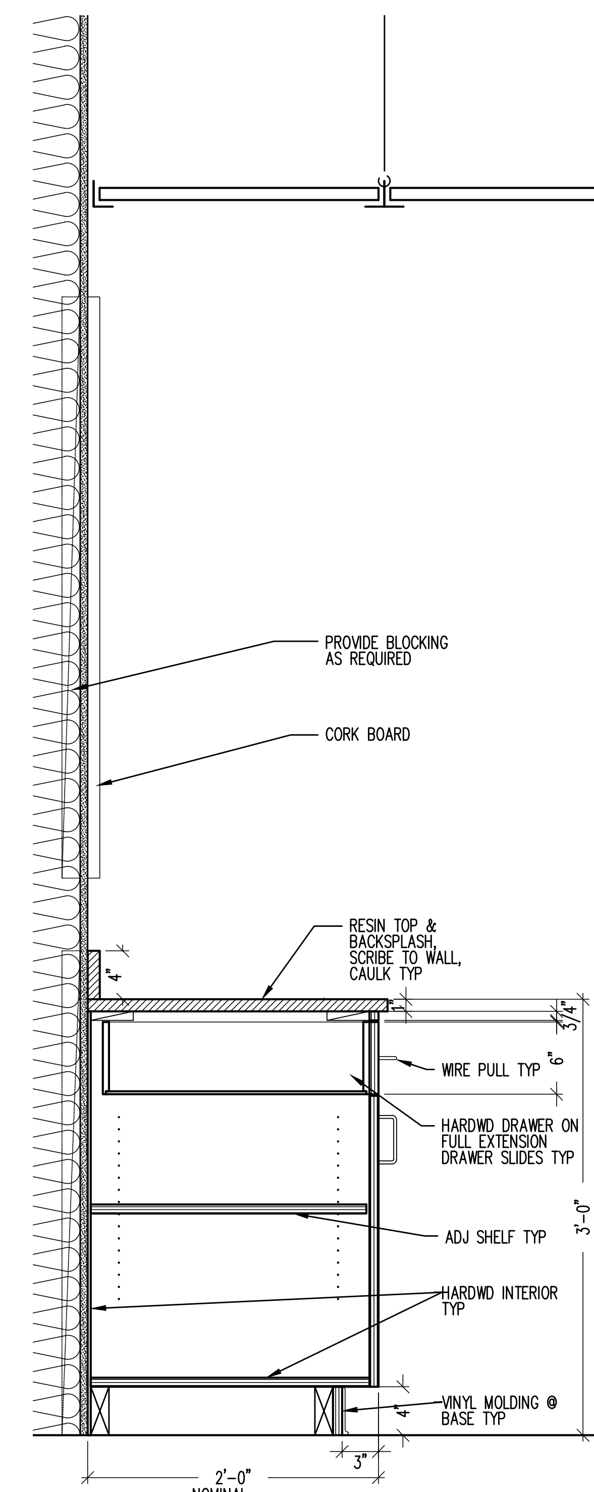
4 SECTION A1.1/A3.1 SCALE: 1-1/2" = 1'-0"
