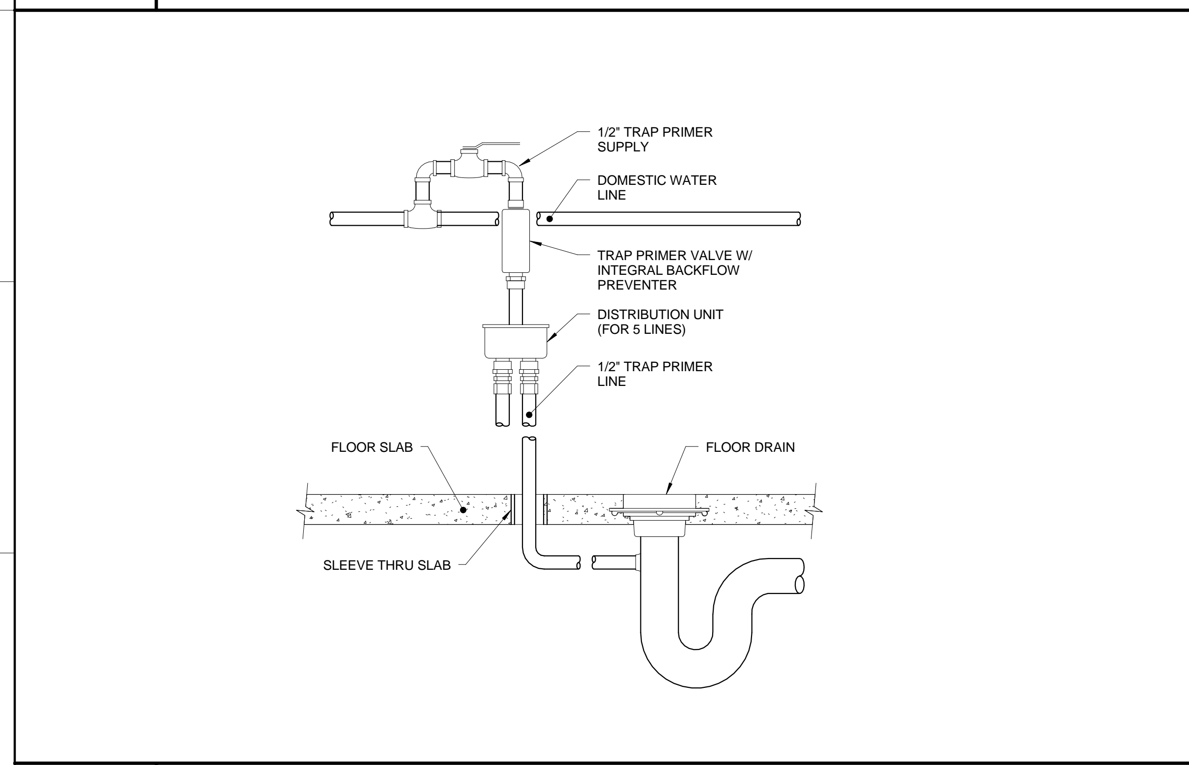
F1 DETAIL - AUTOMATIC TRAP PRIMER
