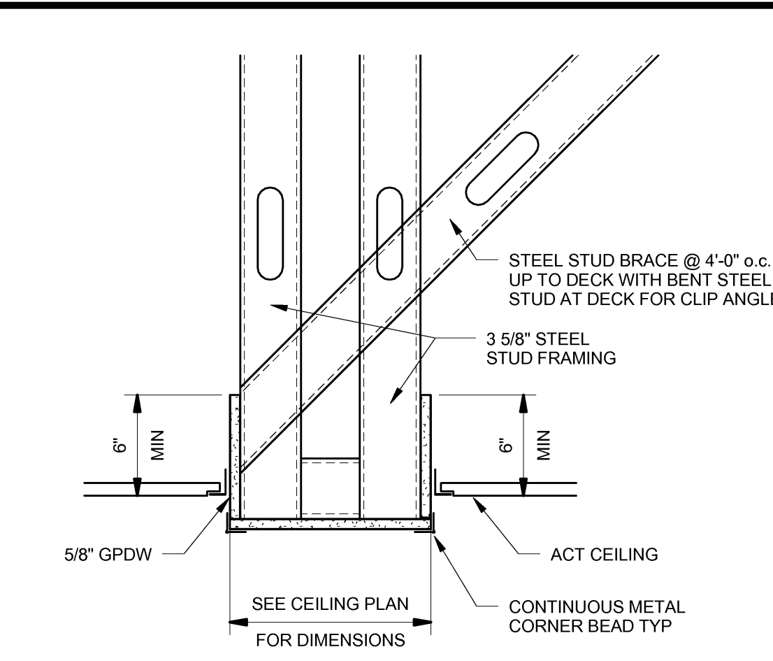
D1 TYPICAL SOFFIT DETAIL SCALE: 1 1/2" = 1'-0"
