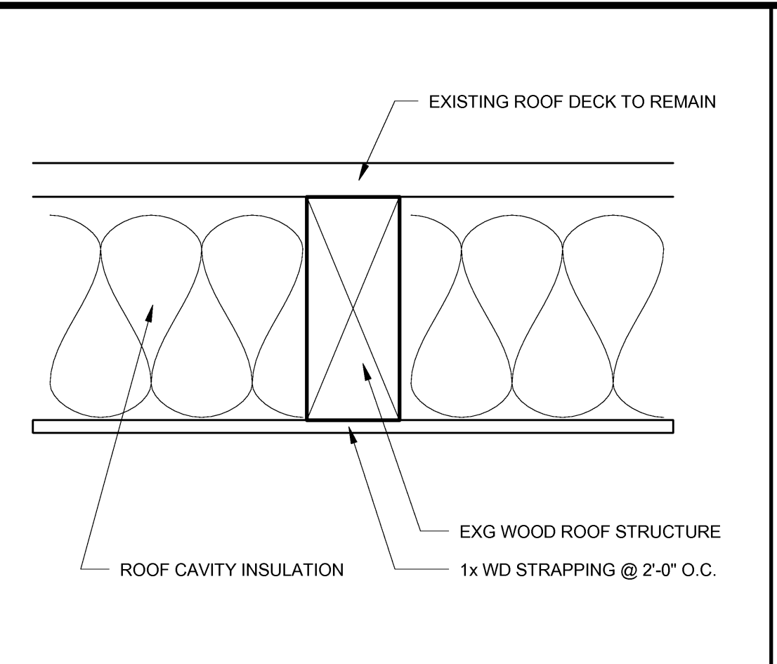
D2 TYP ROOF INSUL INFILL DETAIL SCALE: 1 1/2" = 1'-0"
