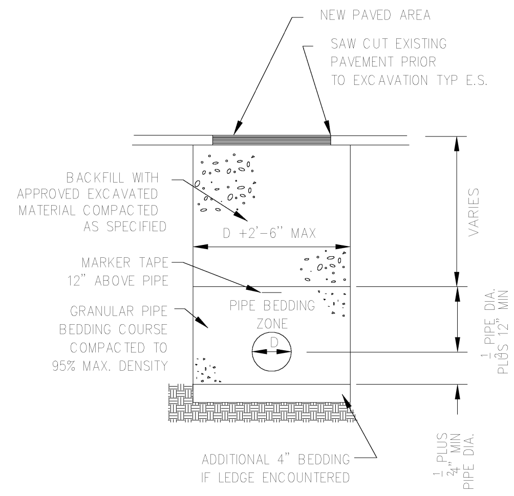
D1 PIPE TRENCH SCALE: 1" = 1'-0"
