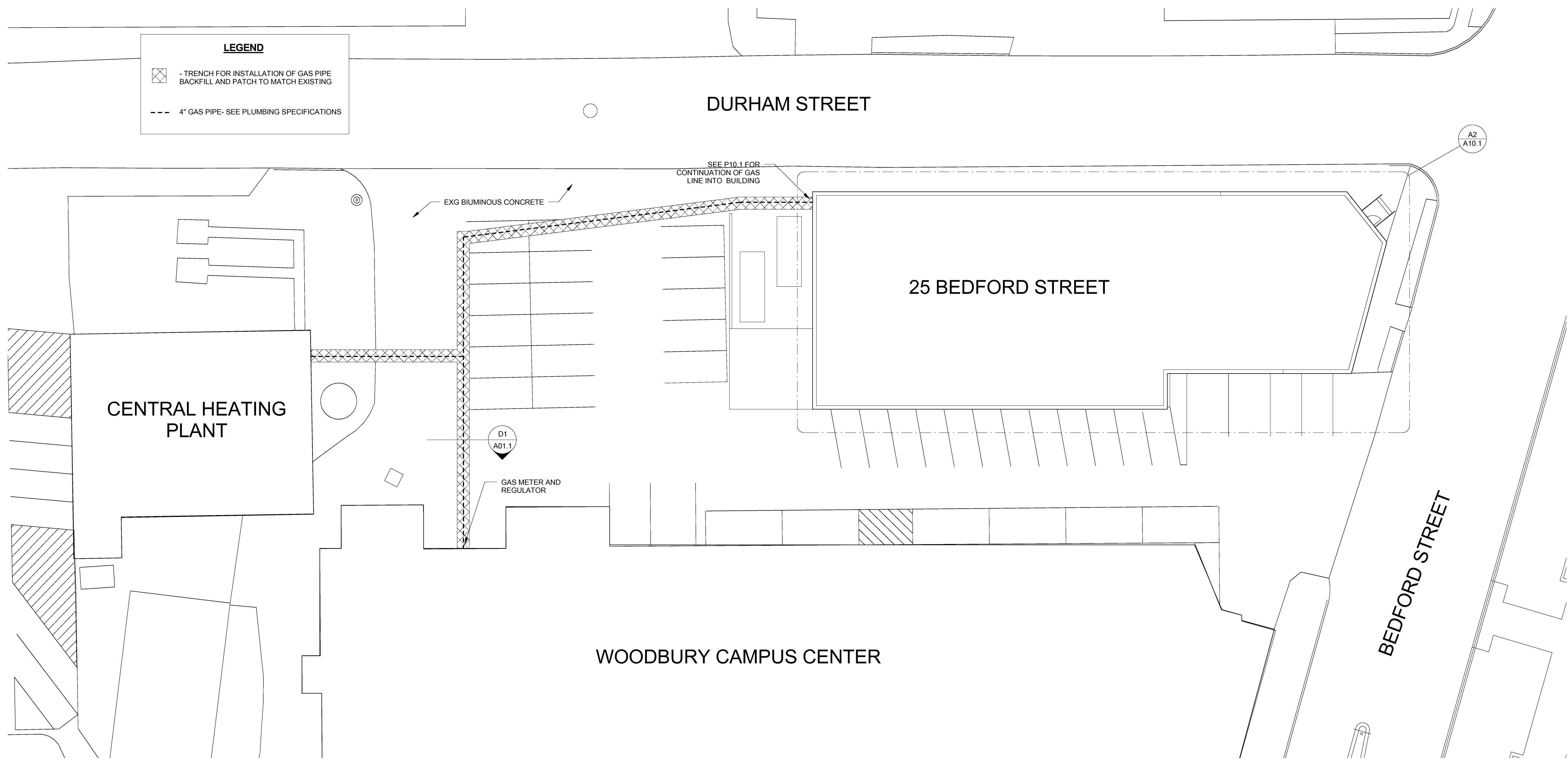
A1 SITE PLAN SCALE: 1/16" = 1'-0"
