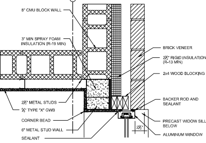
D11 PLAN DETAIL 1:12 = 1:2"
