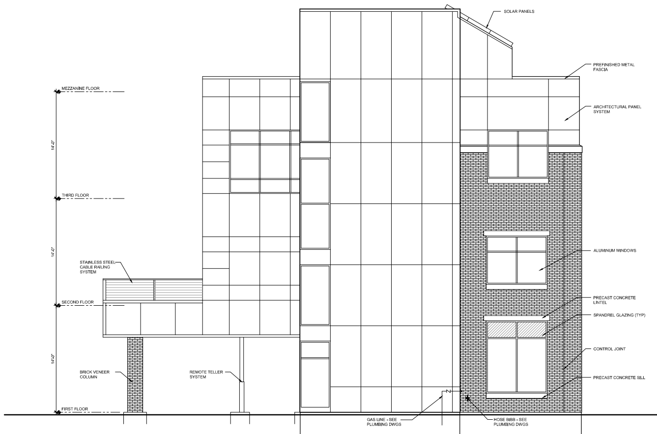
A1 LEFT ELEVATION 1/8" = 1'-0"
