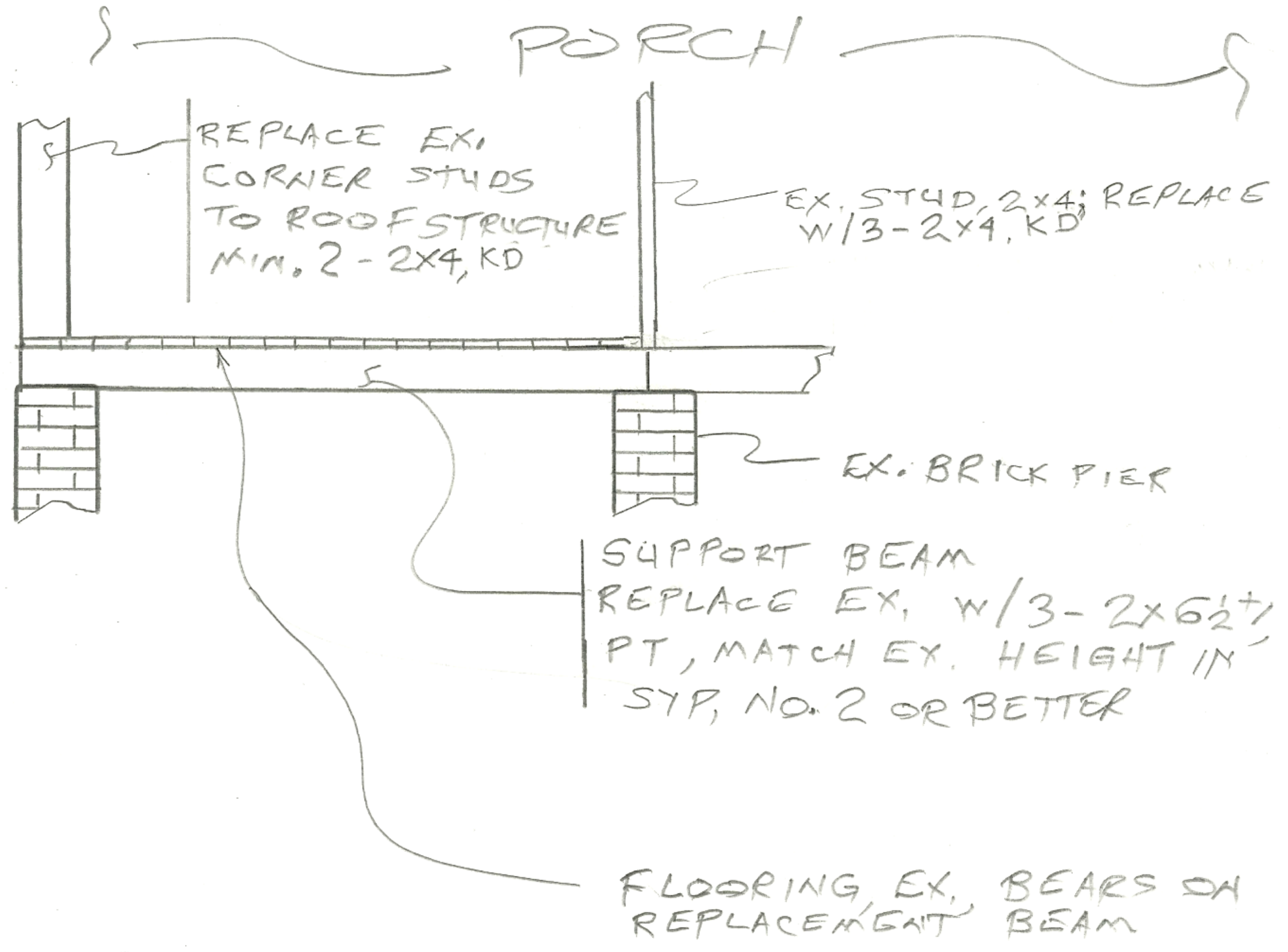
ELEVATION - BACK PORCH N.T.S.
