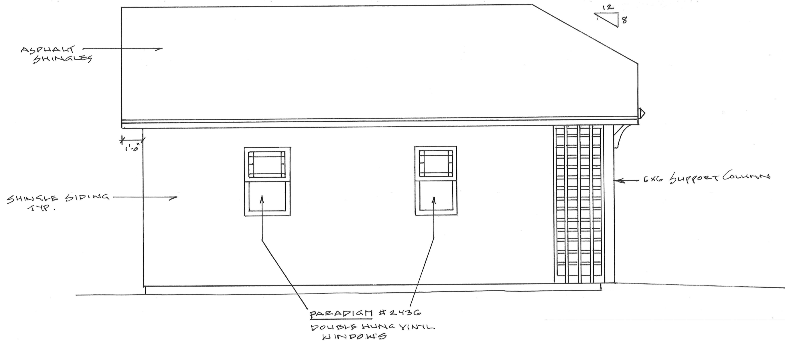
① LEFT SIDE ELEVATION SCALE: 3/8" = 1'-0"
