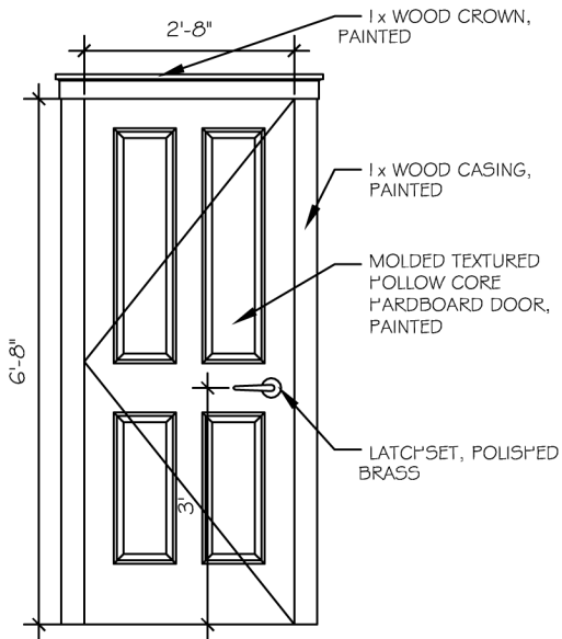
DOOR TYPE A
