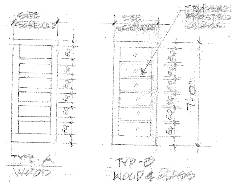
DOOR TYPE & SCHEDULE
