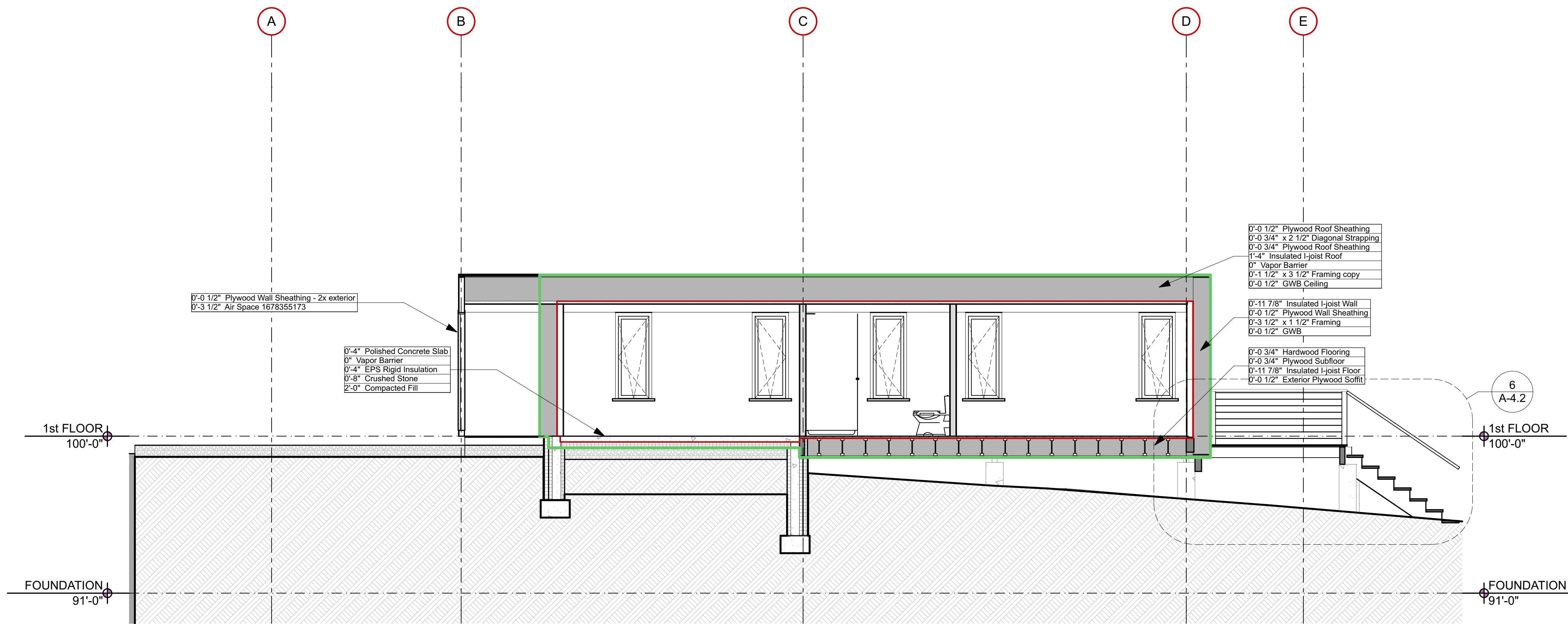
1 LONGITUDINAL-BEDROOMS
