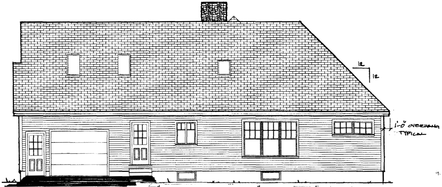
RIGHT ELEVATION
