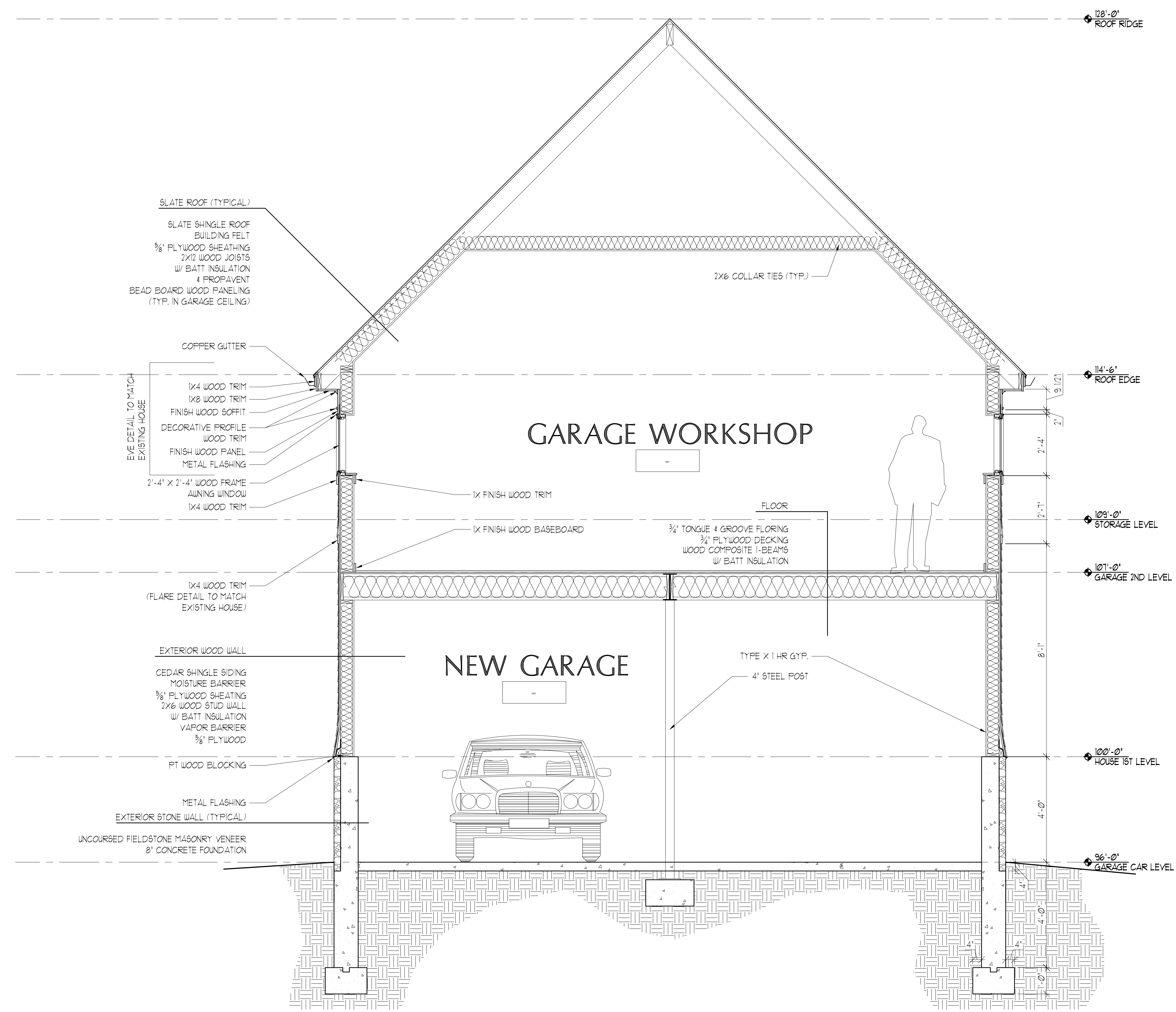
1 SHORT SECTION A1 | A3 | 2'-0" SCALE: 1/2" = 1'-0"
