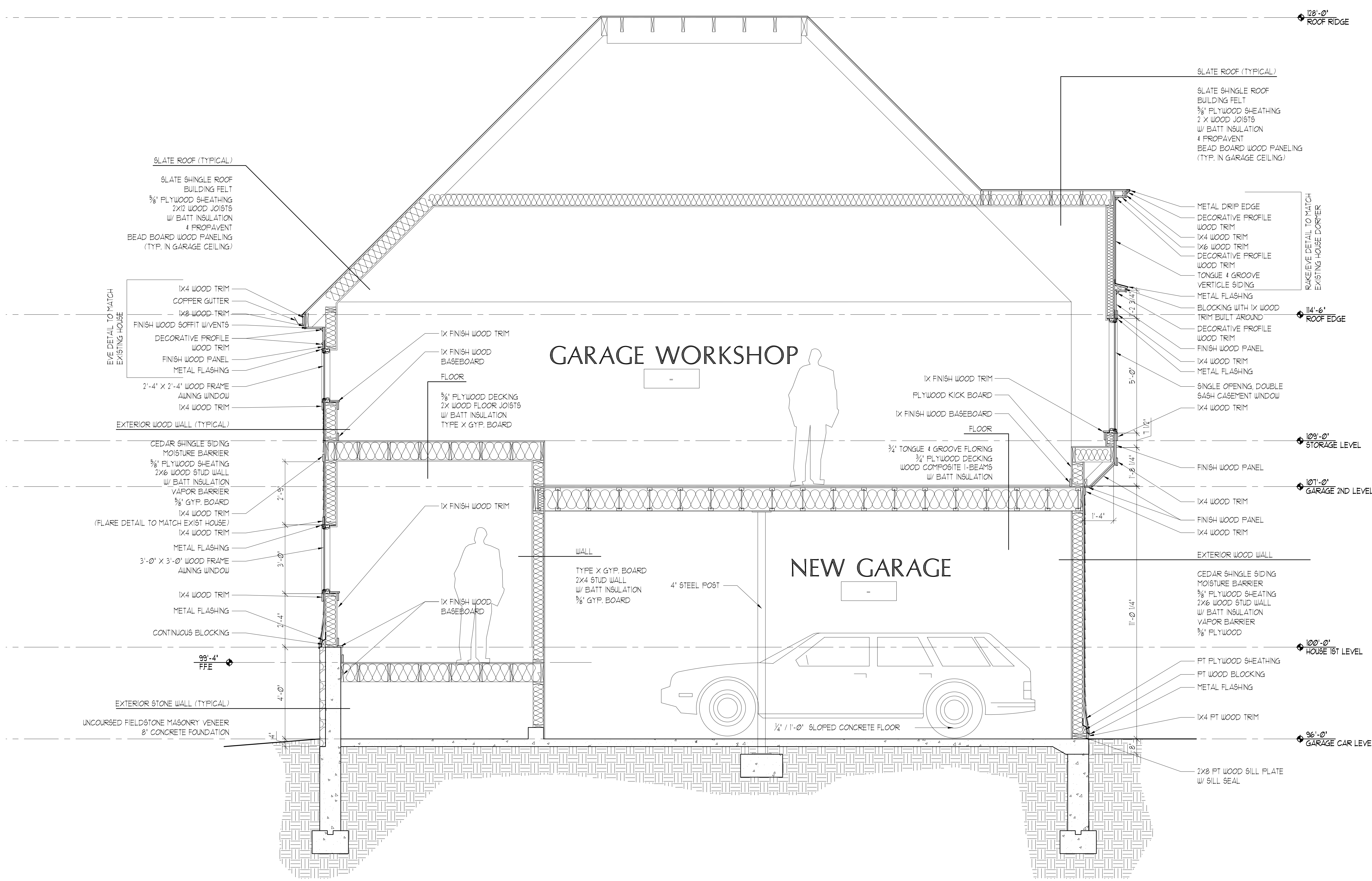
LONG SECTION SCALE: 1/2" = 1'-0"
