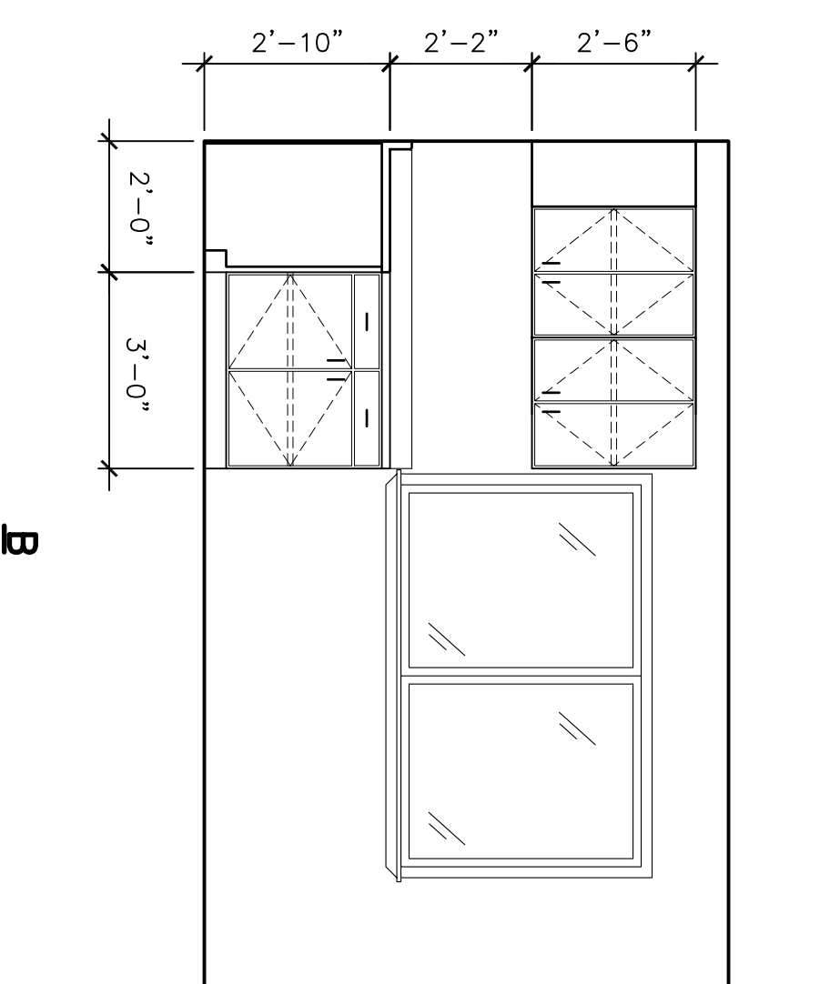
D14 DETAIL
