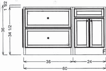
ELEVATION A - DSP
