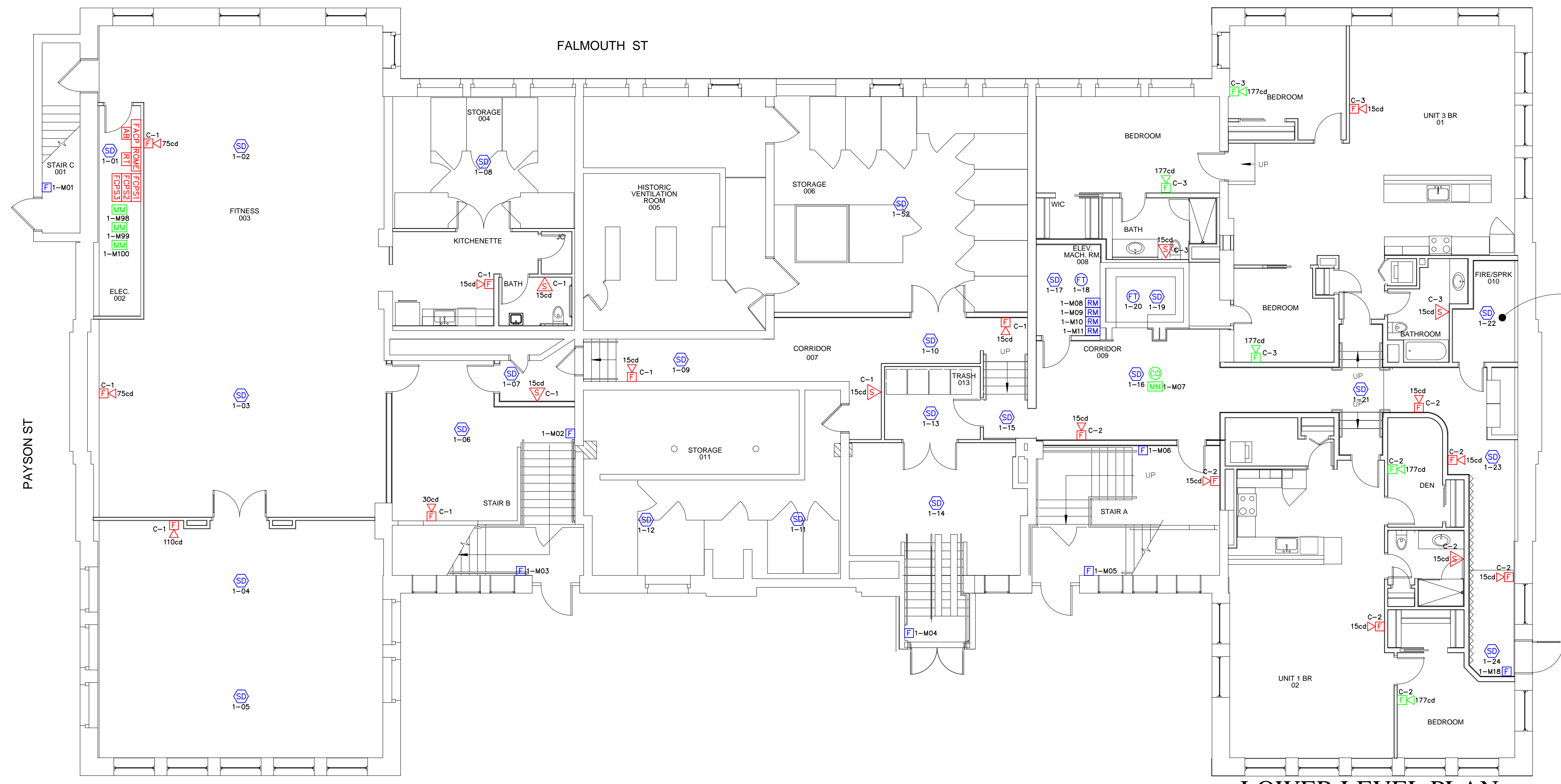
LOWER LEVEL PLAN SCALE: 1/8" = 1'-0"
