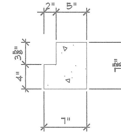
PRECAST HEADER
