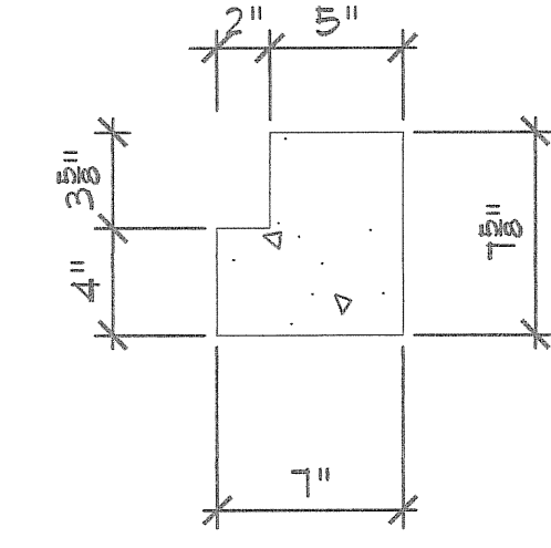
PRECAST JAMB
