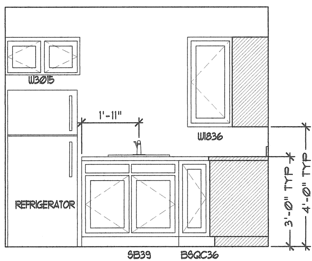
1a ELEVATION SCALE: 1/2" = 1'-0"
