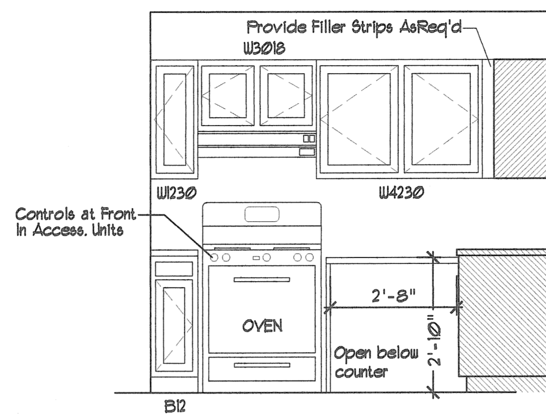
2a ELEVATION SCALE: 1/2" = 1'-0"
