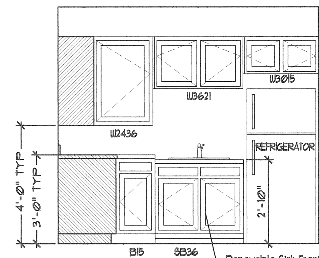
2b ELEVATION SCALE: 1/2" = 1'-0"
