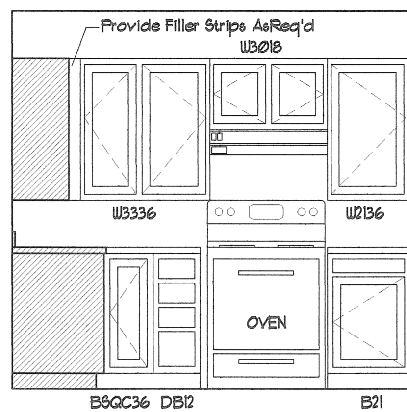
1b ELEVATION SCALE: 1/2" = 1'-0"
