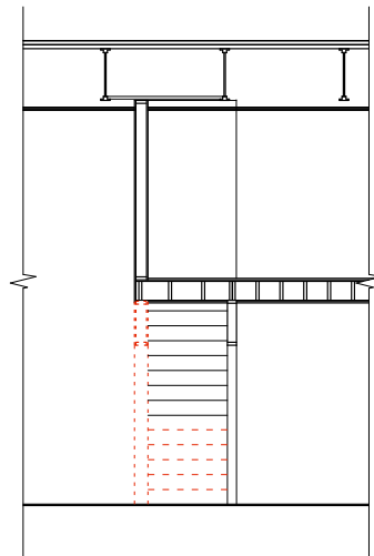
Section CC Demø SCALE: 1/4" = 1'-0"
