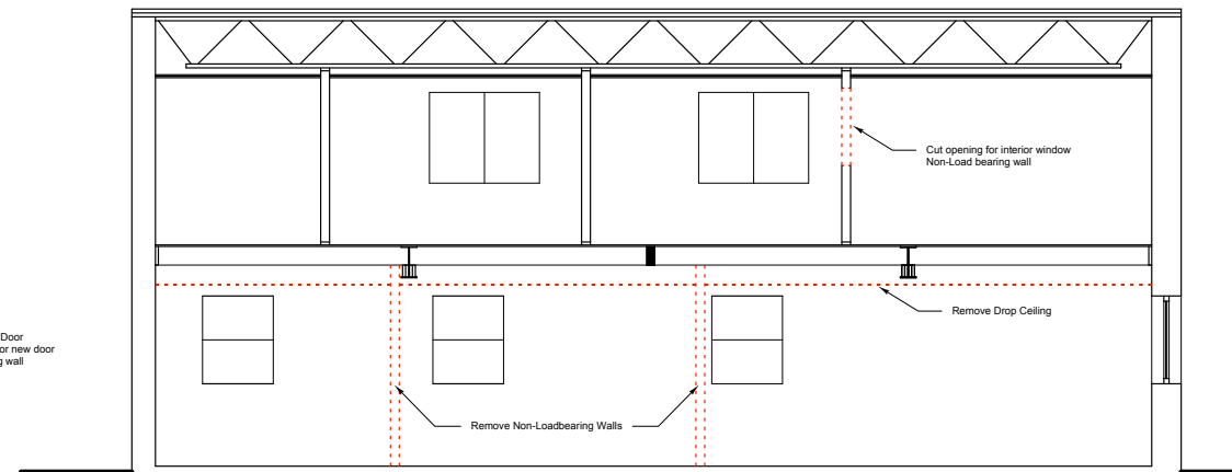
Section BB Demø SCALE: 1/4" = 1'-0"
