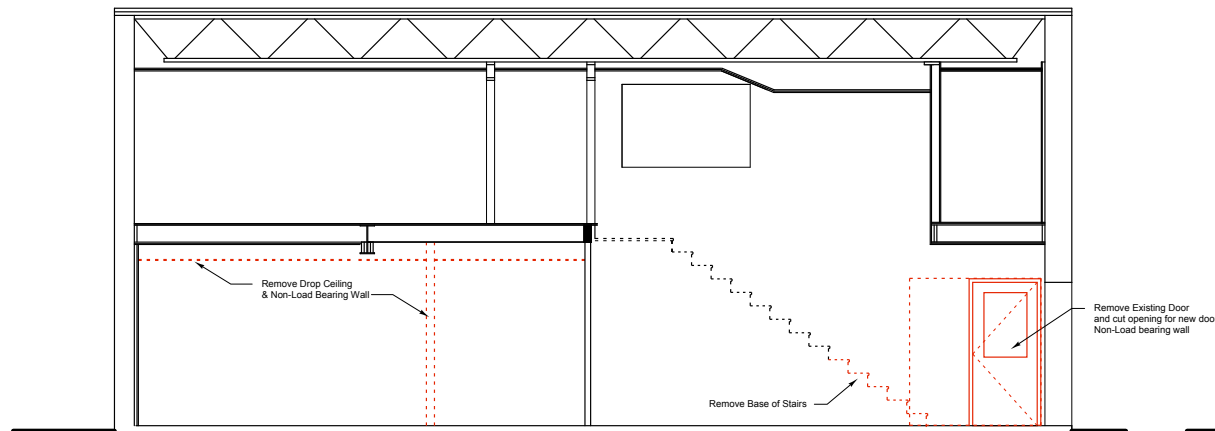
Section AA Demø SCALE: 1/4" = 1'-0"
