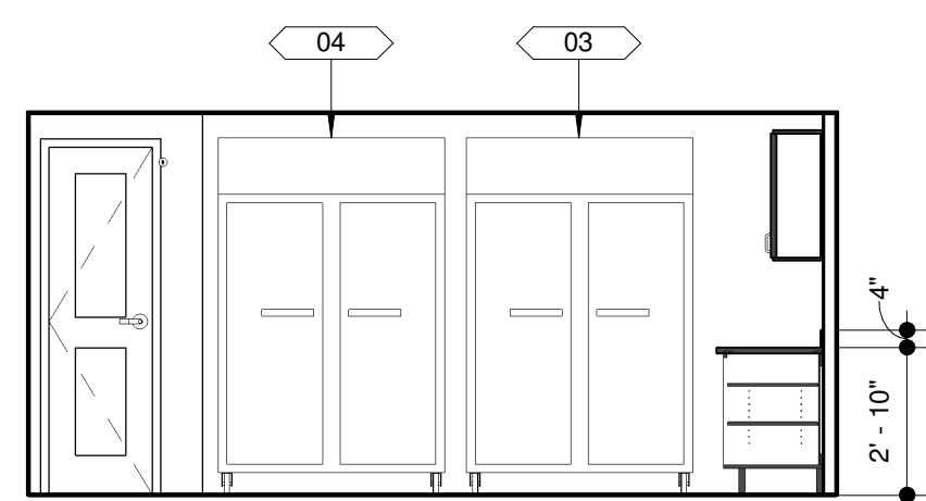
D1 INT. ELEV - KITCHEN - 1 1/4" = 1'-0"
