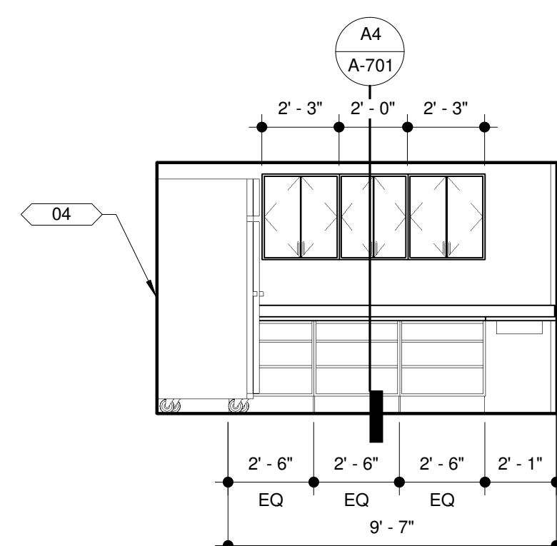
D2 INT. ELEV - KITCHEN - 2 1/4" = 1'-0"
