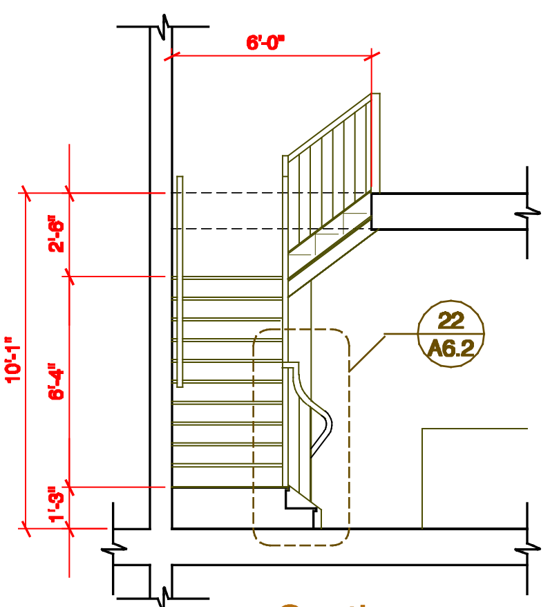
31 Section Scale: 1/4" = 1'-0"
