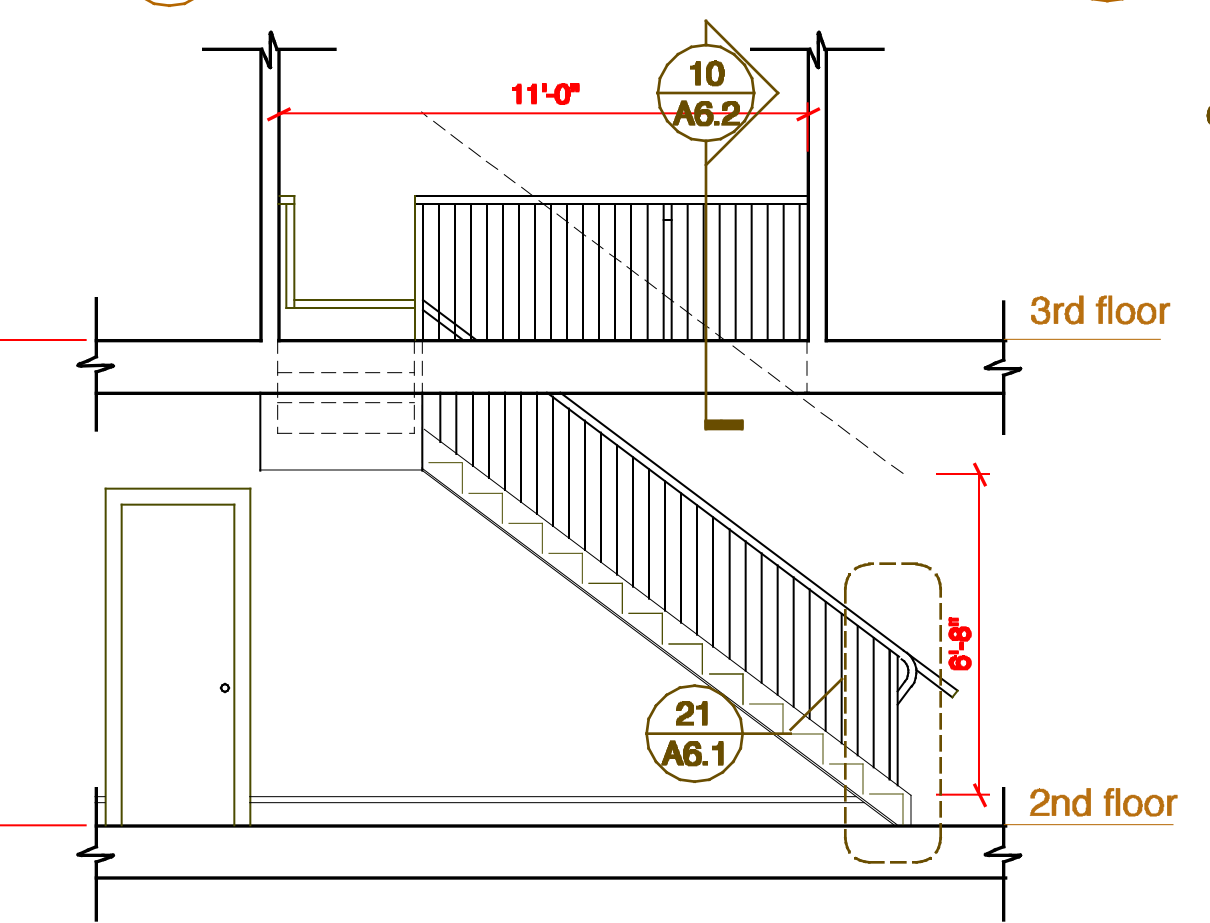
41 Section Scale: 1/4" = 1'-0"
