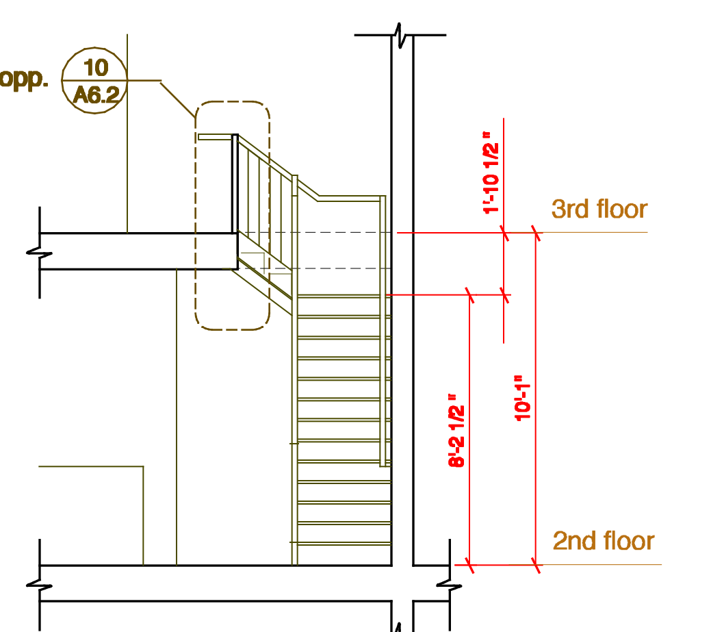
40 Section Scale: 1/4" = 1'-0"
