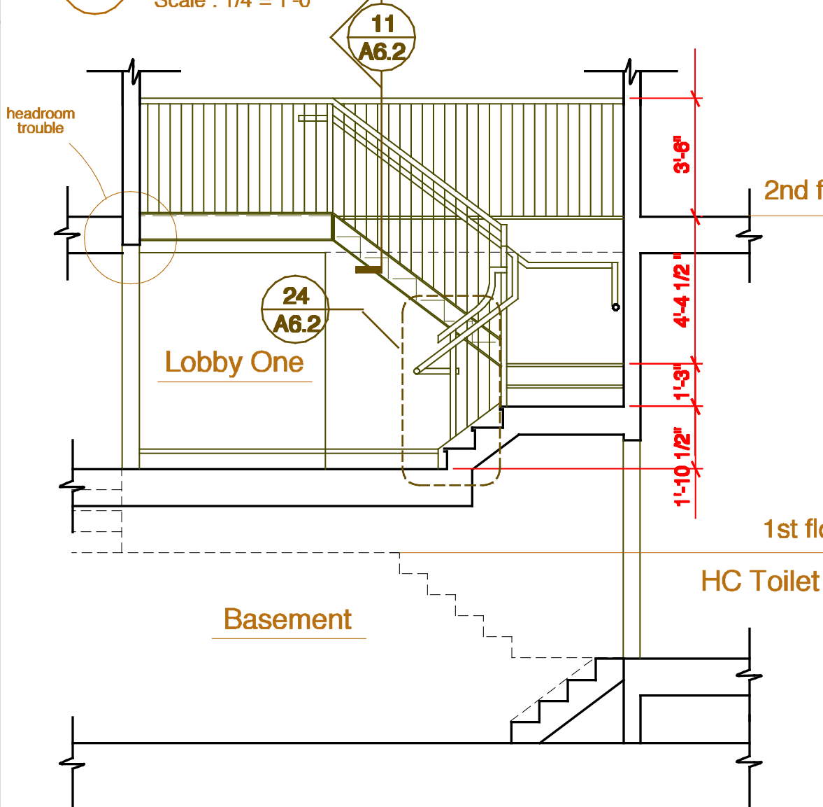
10 Section Scale: 1/4" = 1'-0"
