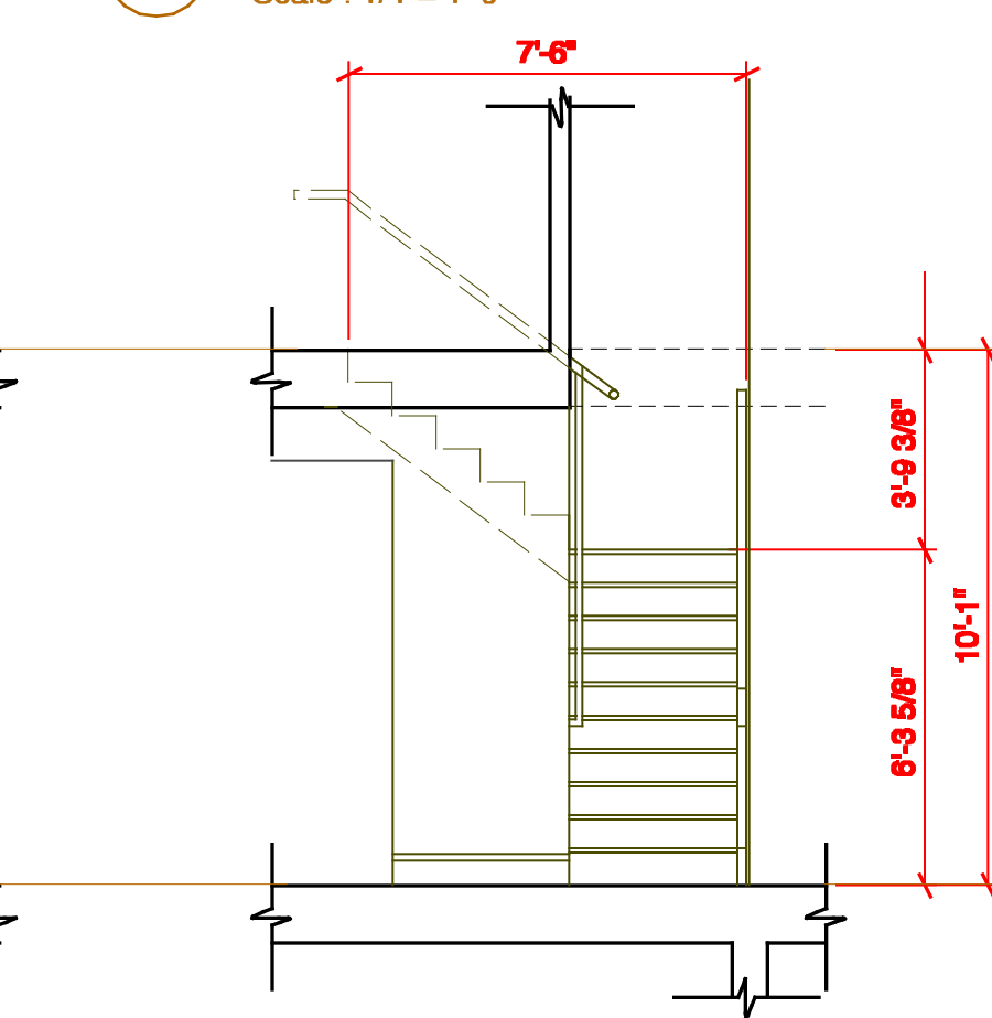
20 Section Scale: 1/4" = 1'-0"
