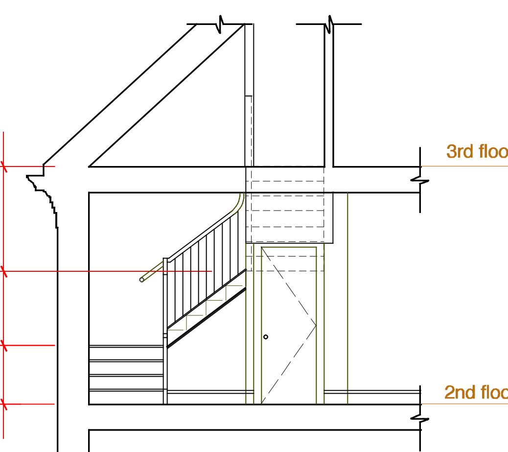
50 Section Scale: 1/4" = 1'-0"
