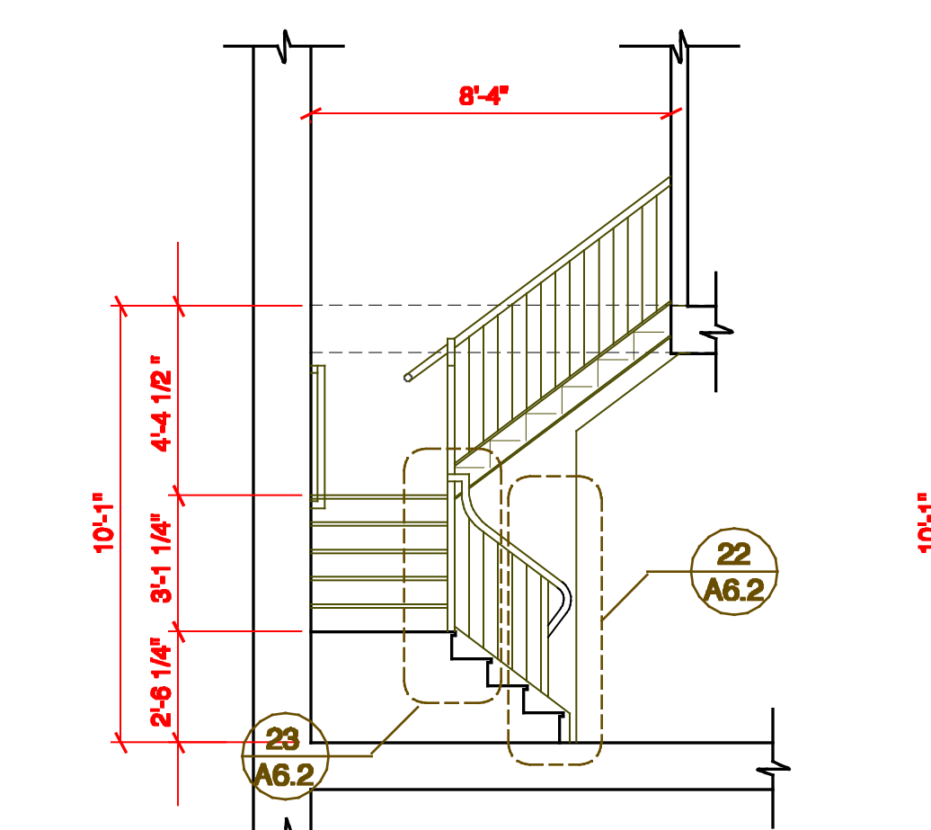
51 Section Scale: 1/4" = 1'-0"
