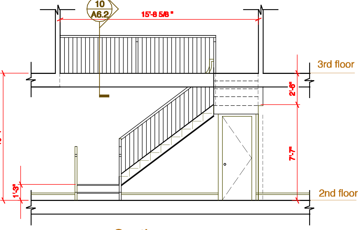
30 Section Scale: 1/4" = 1'-0"
