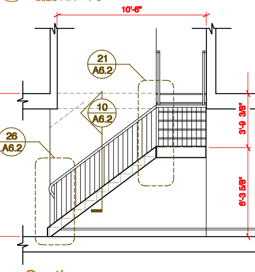
21 Section Scale: 1/4" = 1'-0"
