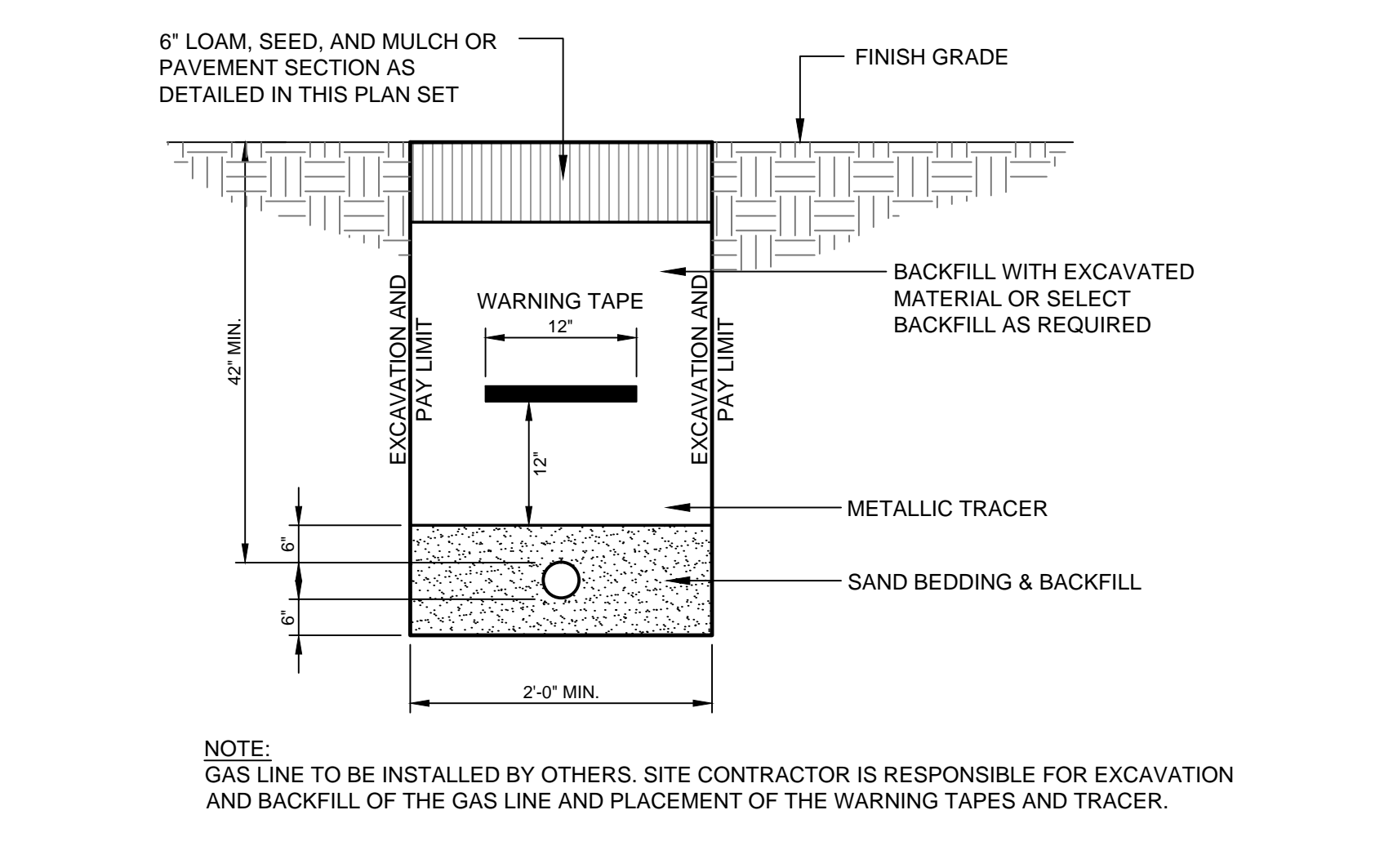
E GAS SERVICE TRENCH SECTION N.T.S.
