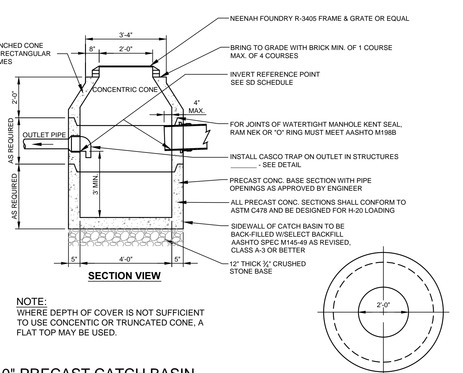
C 4'-0" PRECAST CATCH BASIN N.T.S.
