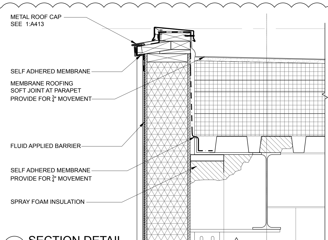
2 SECTION DETAIL SCALE: 1-1/2" = 1'-0"
