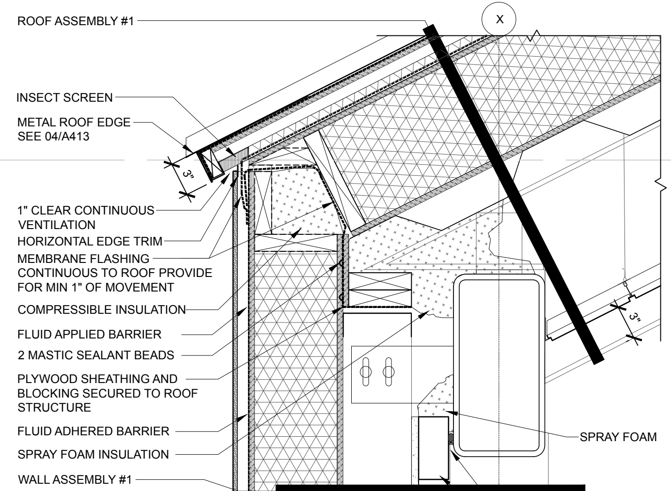
3 SECTION DETAIL SCALE: 1-1/2" = 1'-0"
