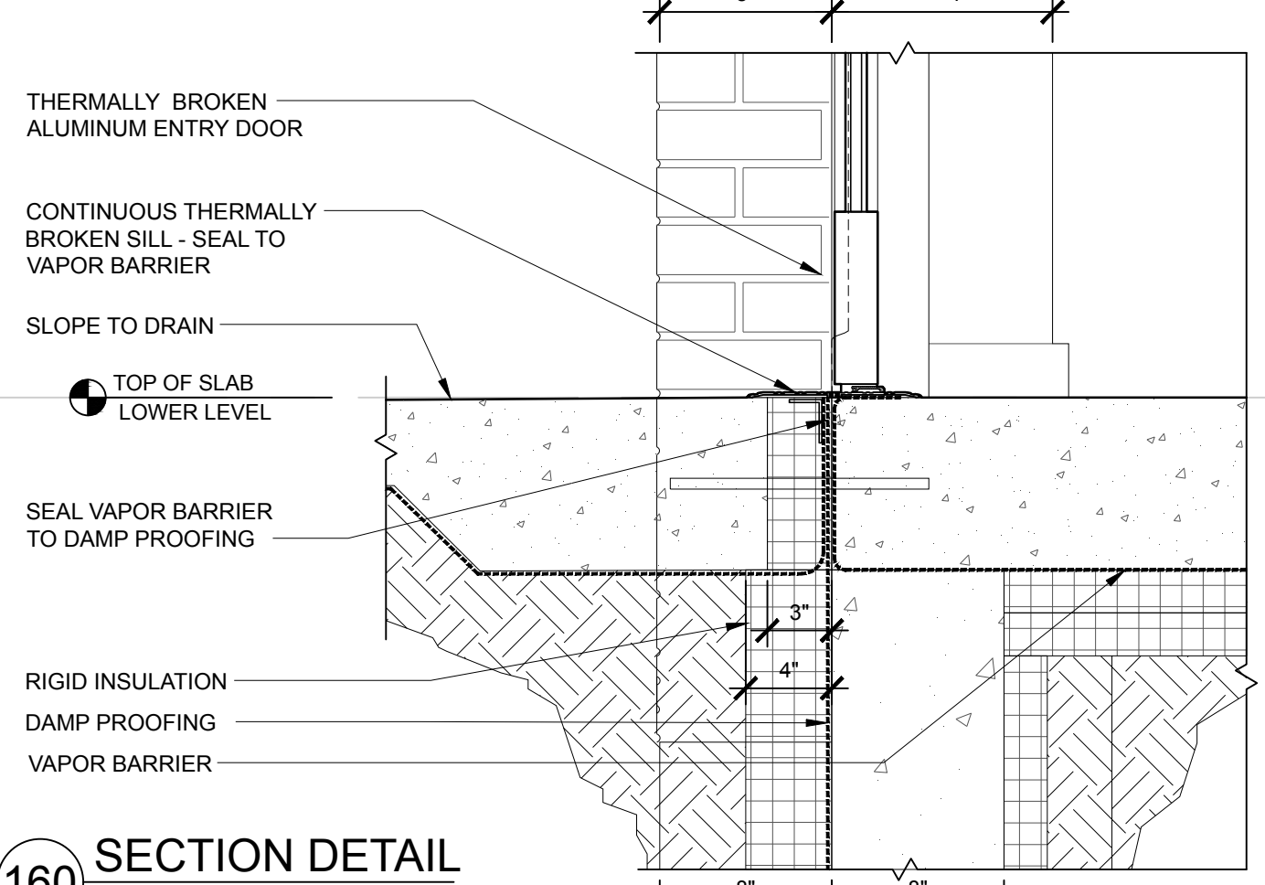
16 SECTION DETAIL SCALE: 1-1/2" = 1'-0"
