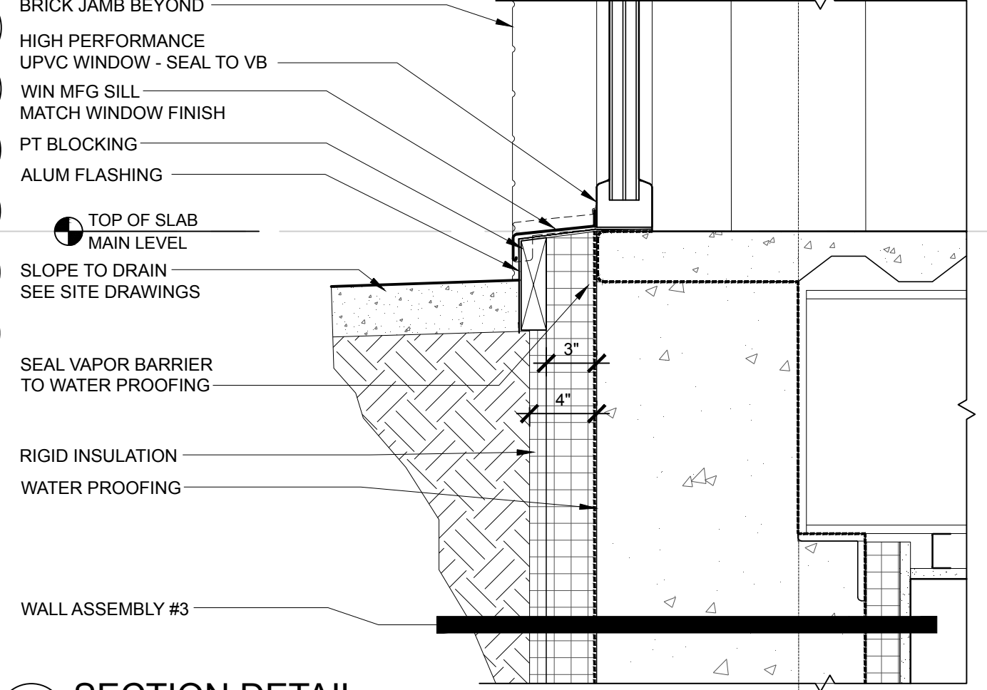
12 SECTION DETAIL SCALE: 1-1/2" = 1'-0"
